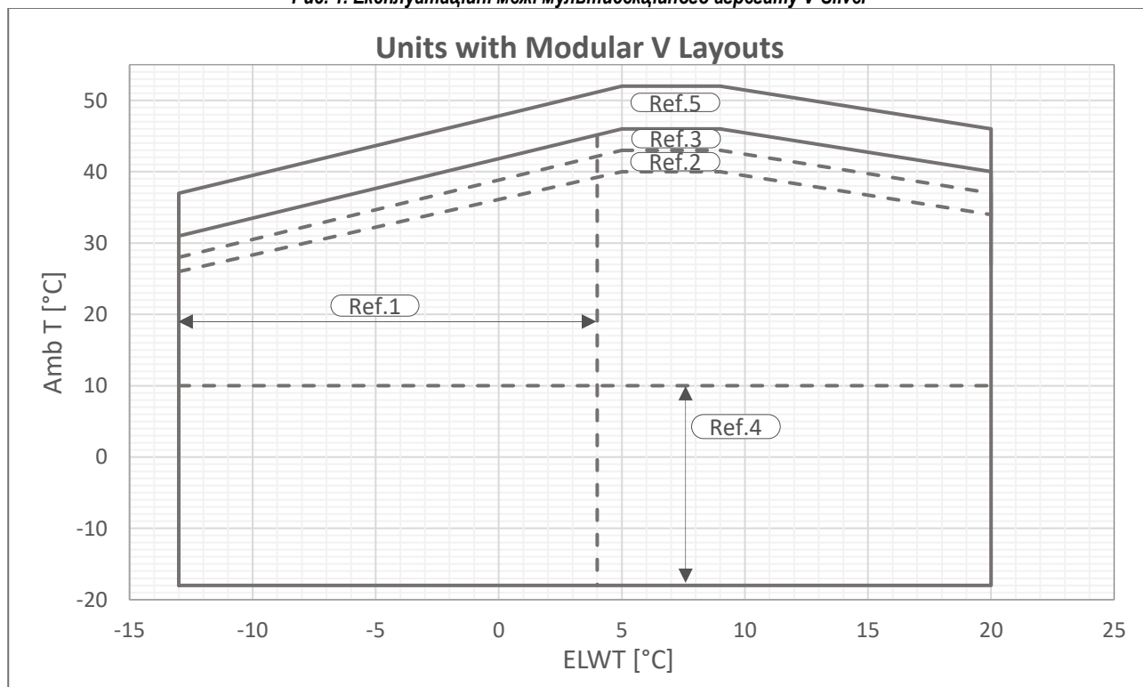
Рис. 2. Експлуатаційні межі мультисекційного агрегату V-Gold
