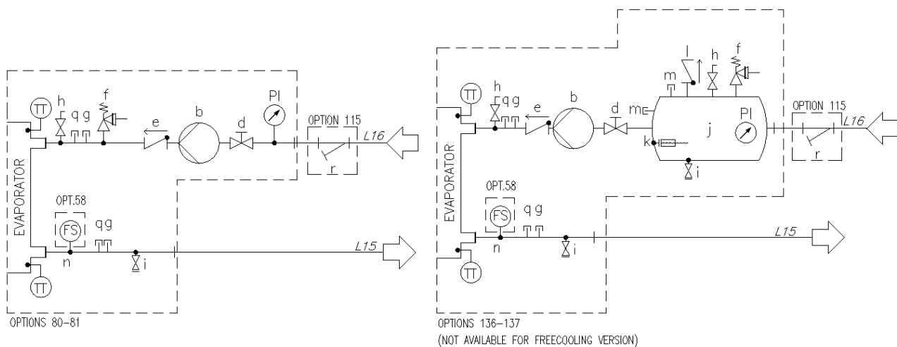
Рис. 11. Гідравлічна схема односекційного агрегату (EWATxx5B) зі здовжнім насосом (компл. 80-81/136-137) (макс. робочий тиск 6 бар)
