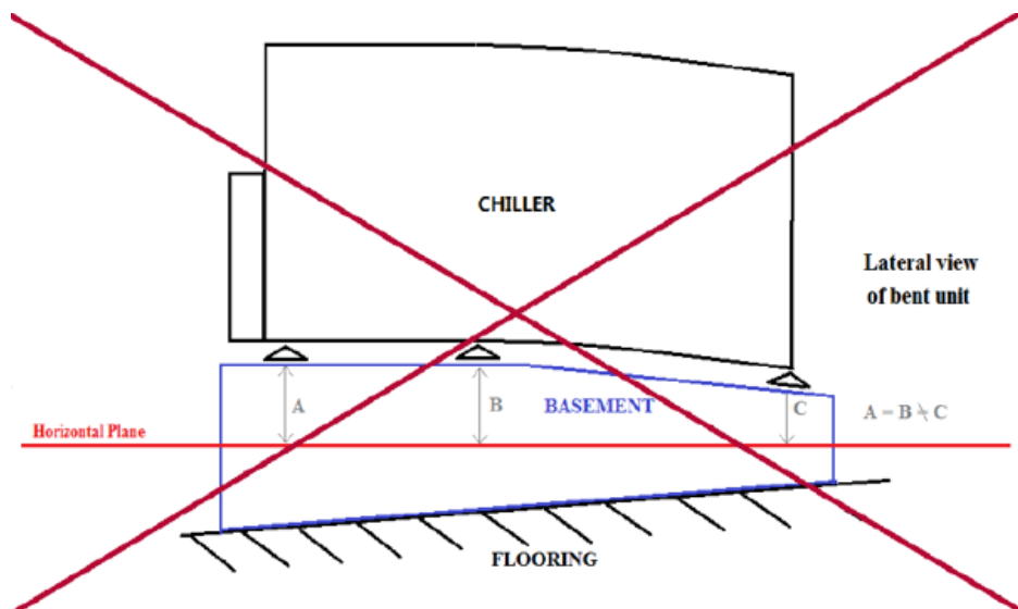
Рис. 6. Вирівнювання агрегату
