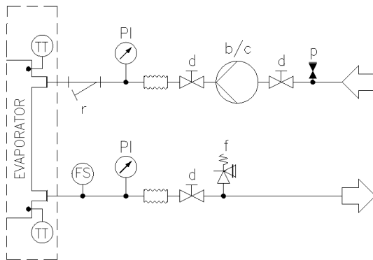
Рис. 9. Гідравлічна схема агрегату без вбудованого насоса (макс. робочий тиск 20 бар)
