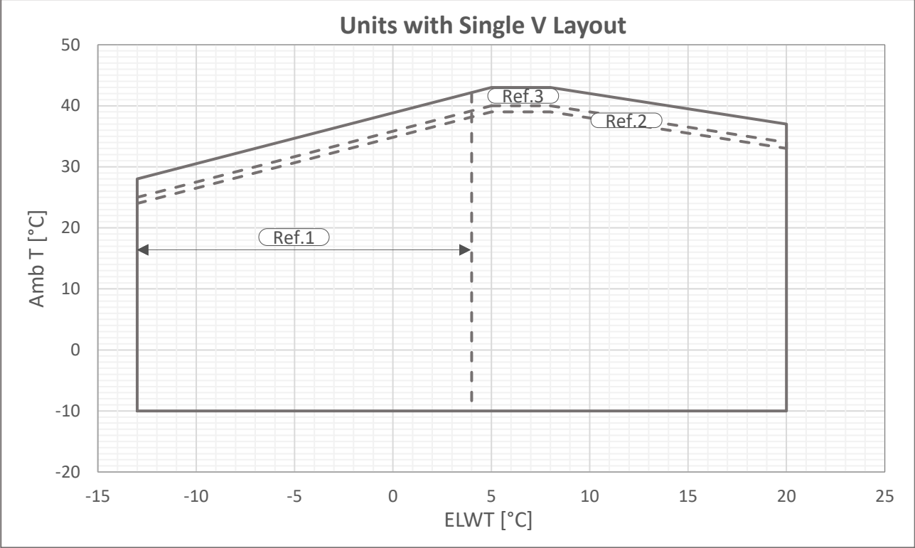
Рис. 3. Експлуатаційні межі одnoseкційного агрегату V-Silver
