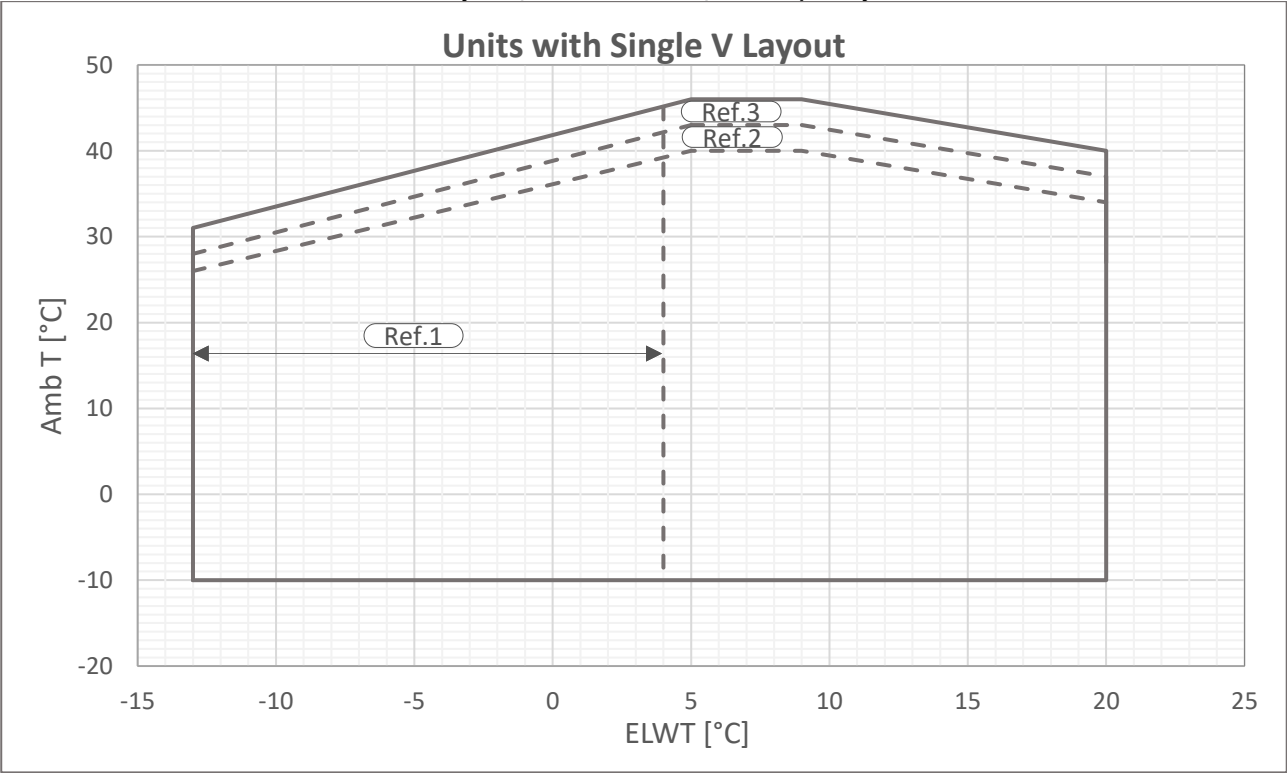
Рис. 4. Експлуатаційні межі одnoseкційного агрегату V-Gold
