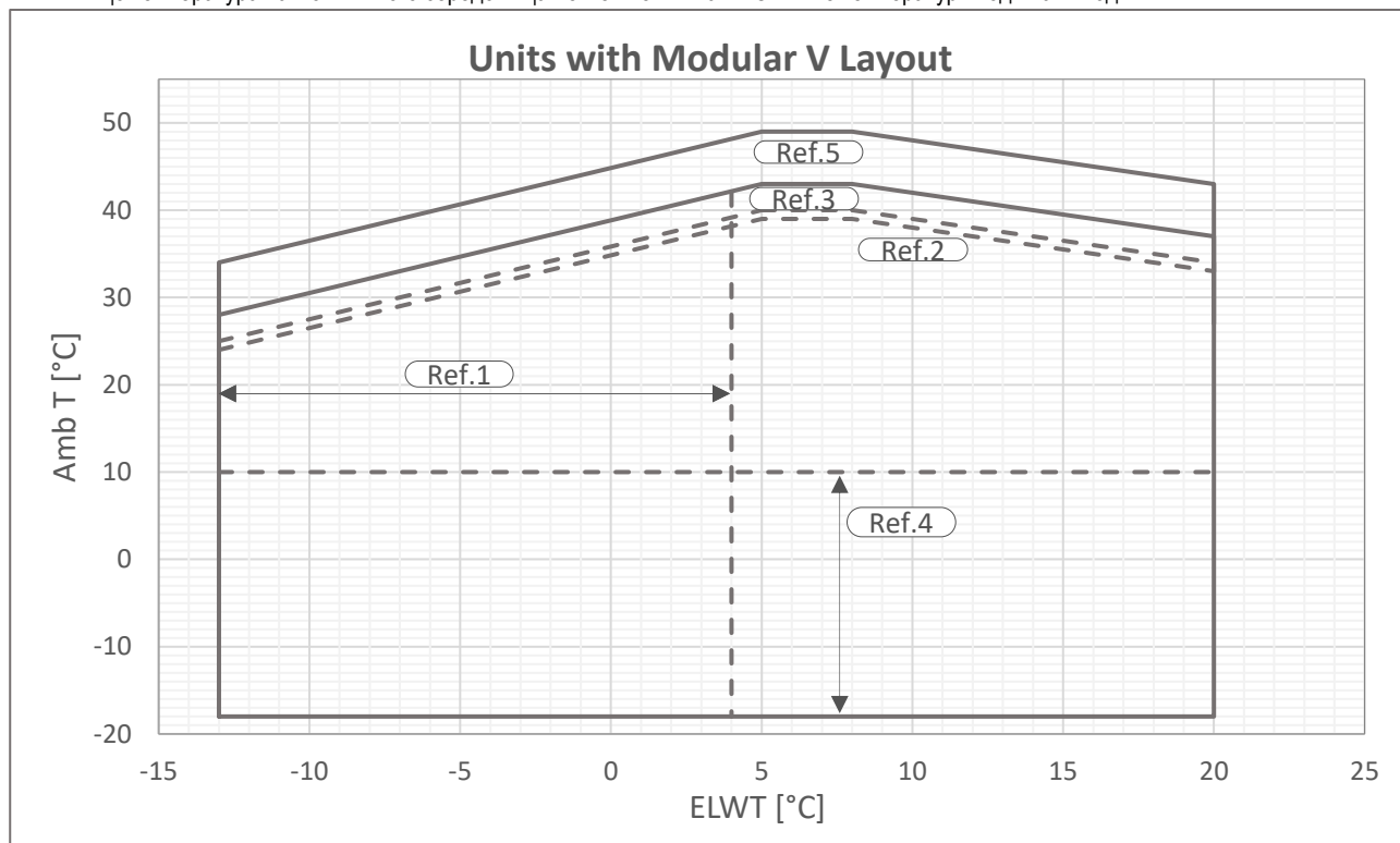
Рис. 1. Експлуатаційні межі мультисекційного агрегату V-Silver
