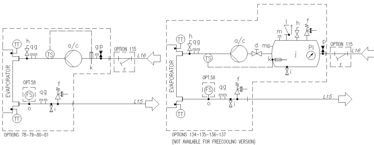
Рис. 12. Гідравлічна схема мультисекційного агрегату (EWATxx0B) (компл. 78-79-80-81/134-135-136-137) (макс. робочий тиск 6 бар)
