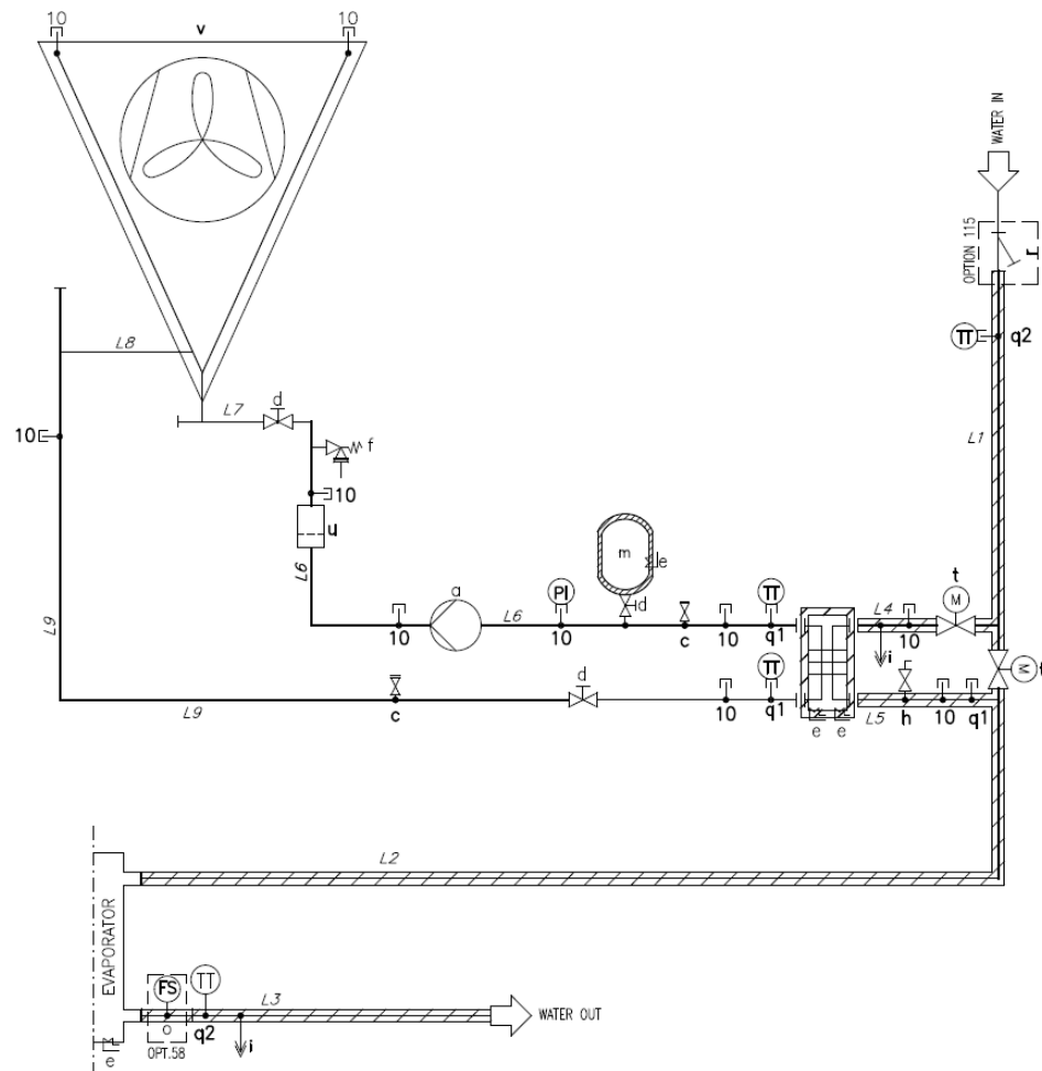
Joonis 26 - suletud ahelaga hüdrooniline vabajahutus P&ID (Opt. 231)
