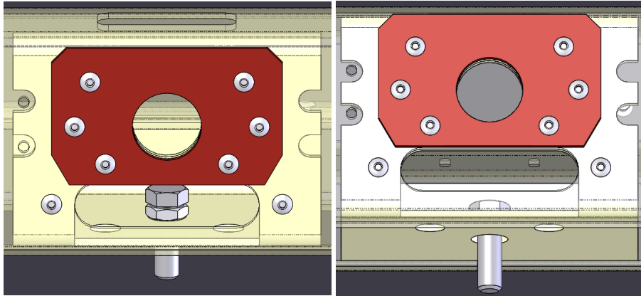
Joonis 21- Vibratsioonivastase summuti kinnituskruvi detail
