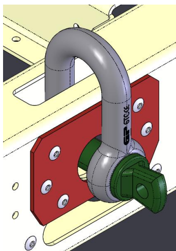
Kuva 12- Nostokahvojen asennus
