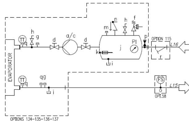
Kuva 24- Hydraulikaavio (lisävaruste 78-79-80-81/134-135-136-137)
