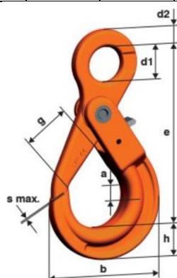
Kuva 9- Nostokoukun ominaisuudet
