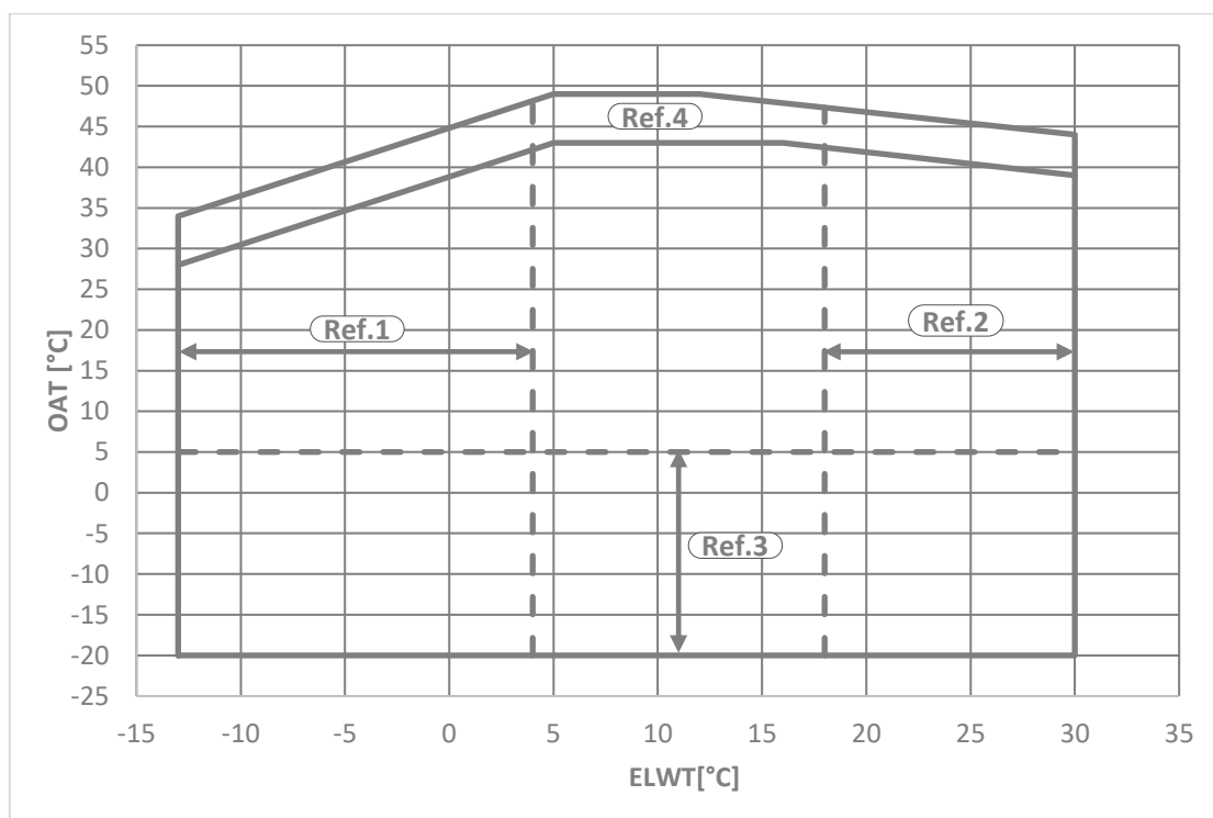
4. ábra – EWAT-B-C Silver egység üzemi tartományai
