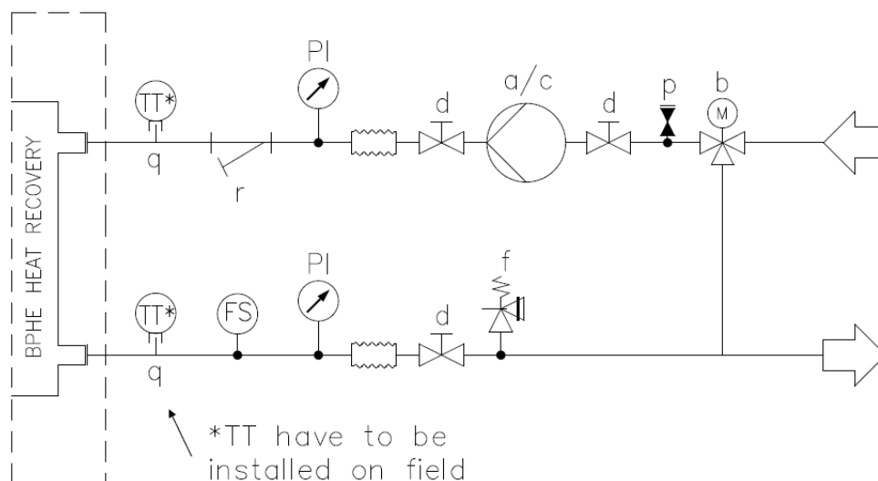
19. ábra - Vízvezeték-csatlakozás hővisszanyerős hőcserélőkhöz (maximális nyomás: 20 bar)
