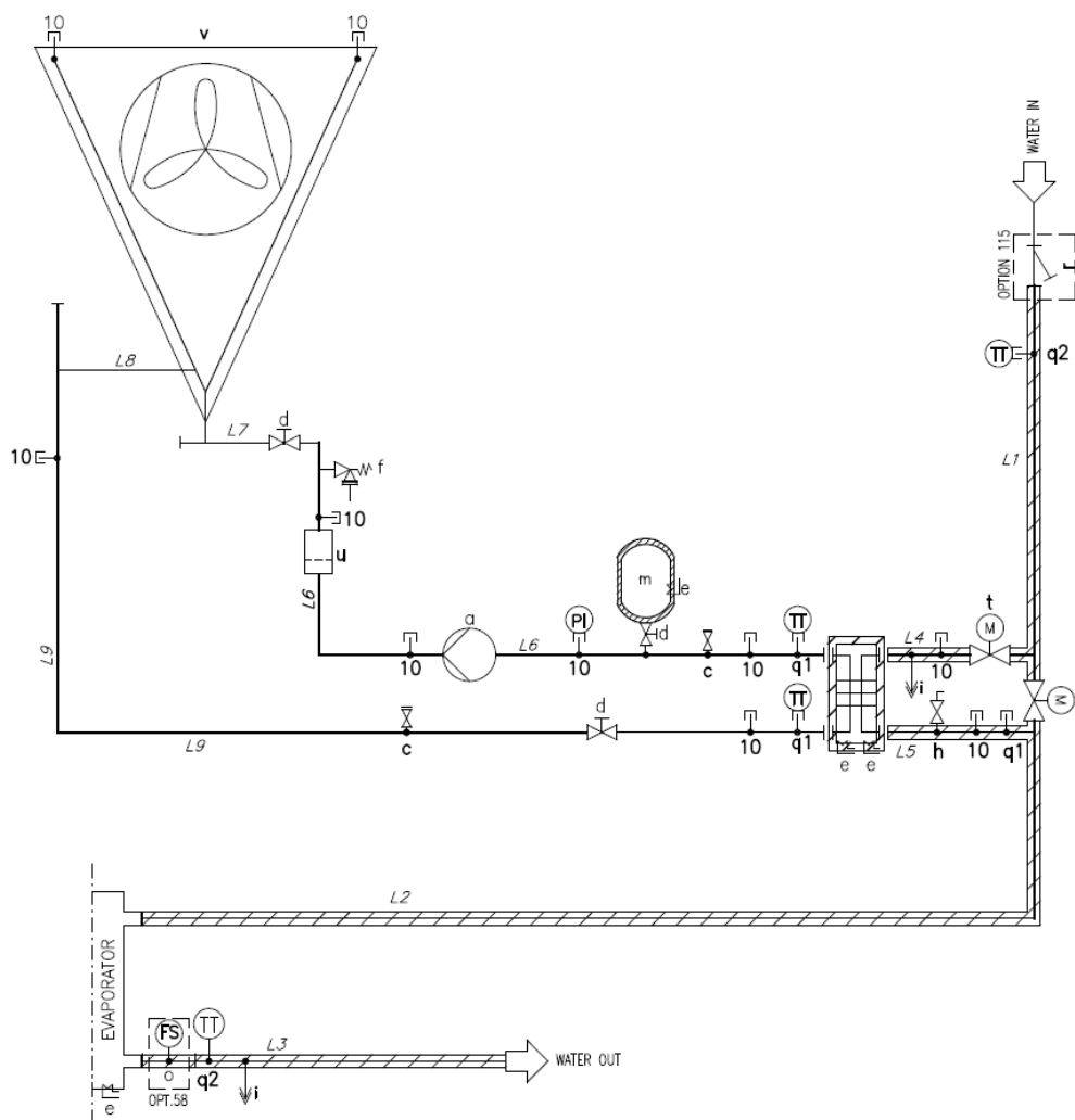
20. ábra – Zárt hurok Hydronic Ingyenes hűtés P&ID (Opt. 231)
