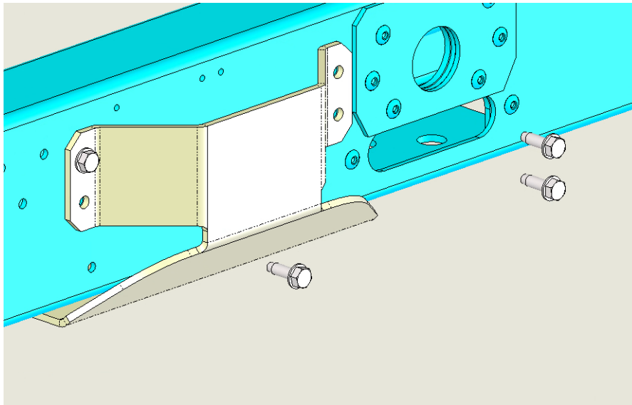
11. ábra – M8 csavarok a lemezegység keretének csatlakoztatásához
