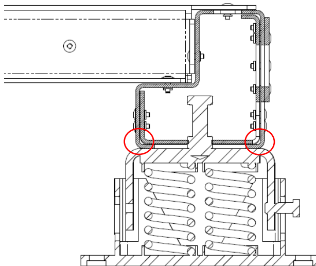
17. ábra: Rezgéscsillapító elemek felszerelése (opcionális)
