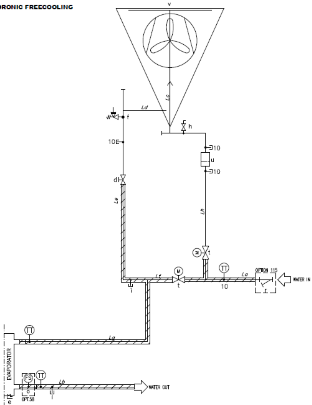
3. ábra: Vízkör diagramja (P&ID) hidronikus szabadhűtéses rendszer
