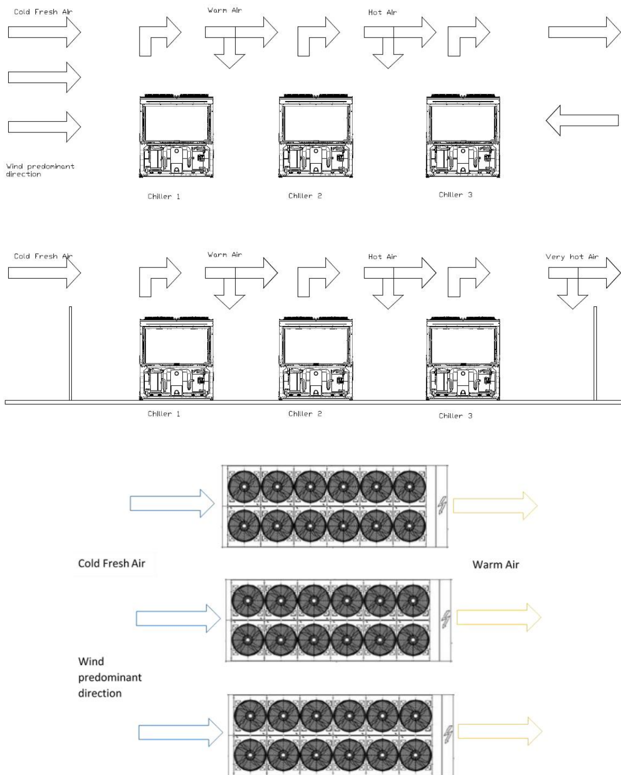
Fig. 17– Installation av flera kylare
