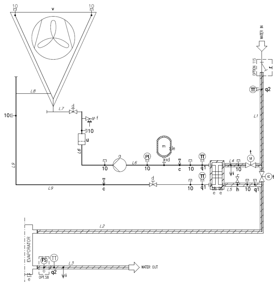
Fig. 26- Hydronisk frikyla med sluten krets P&ID (Opt. 231)
