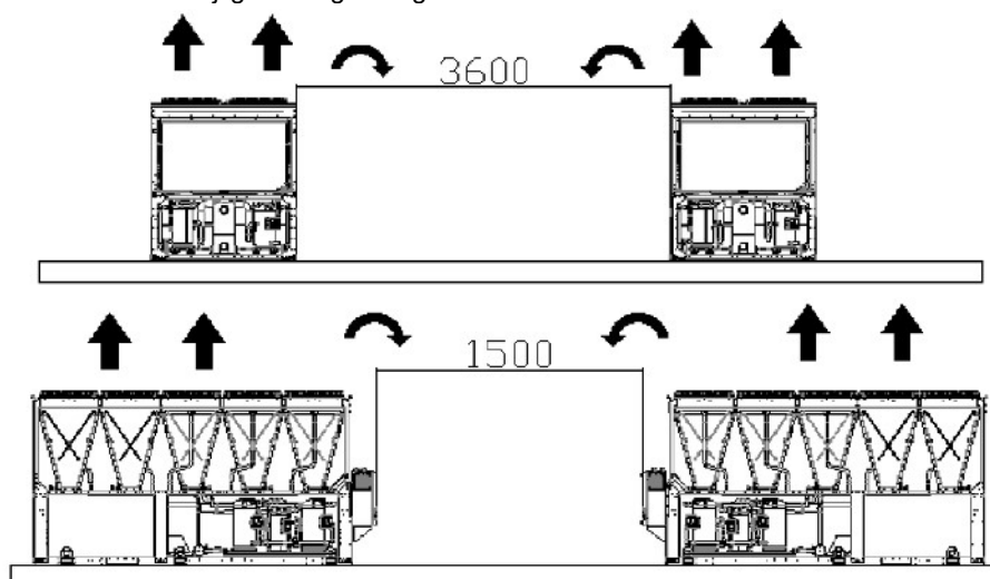
Fig. 16– Krav på minsta utrymme
