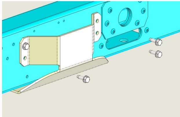
Fig. 22 – Boulons M8 pour le raccordement des plaques au châssis de l'appareil
