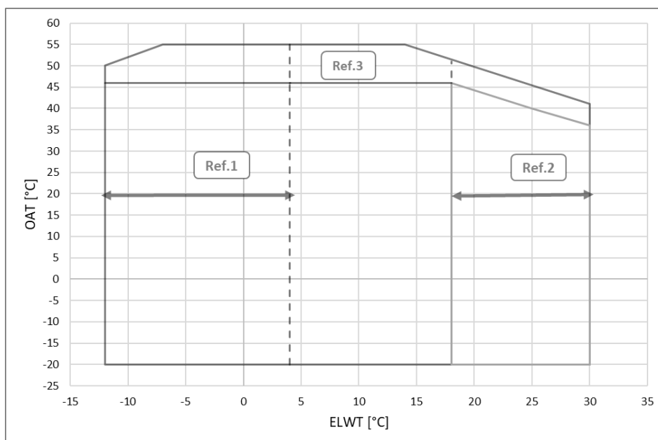
Fig. 13 – EWFH-TZD enveloppe unité Blue et Silver
