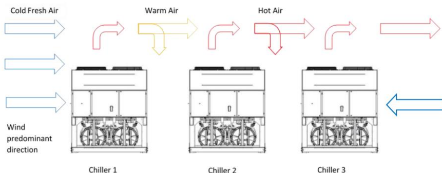
Fig. 26 – Installation de refroidisseurs multiples
