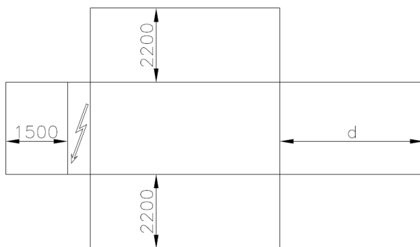
Fig. 25 - Encombrement minimal
