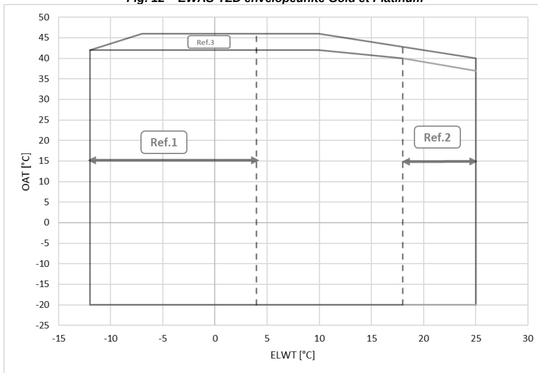
Fig. 12 – EWAS-TZD enveloppe unité Gold et Platinum
