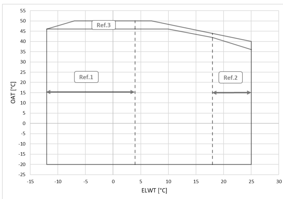
Fig. 15 – EWFD-TZD envelope Blue et Silver
