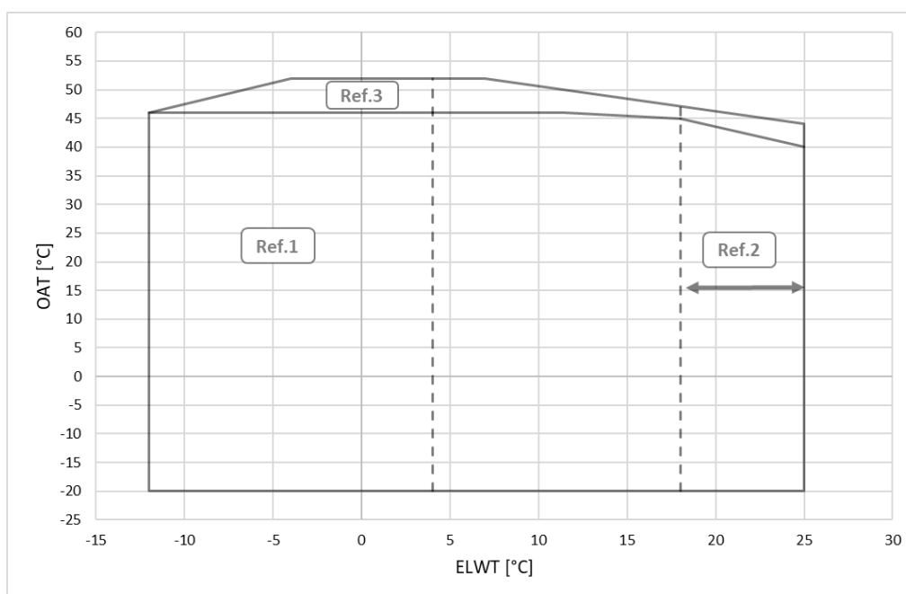
Fig. 9 – EWAD-TZD envelope unité Gold et Platinum
