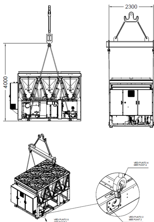
Fig. 18 – Instructions de levage
