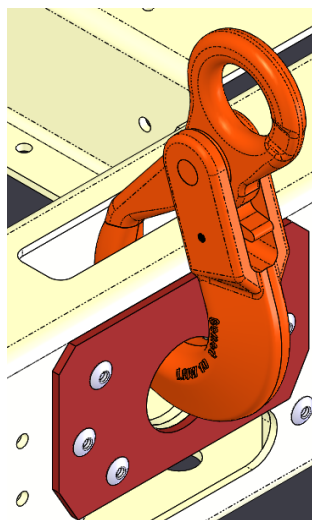
Fig. 19 - Fixation du crochet de sécurité
