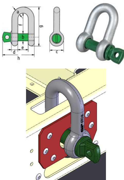
Fig. 20 - Fixation des manilles de levage
