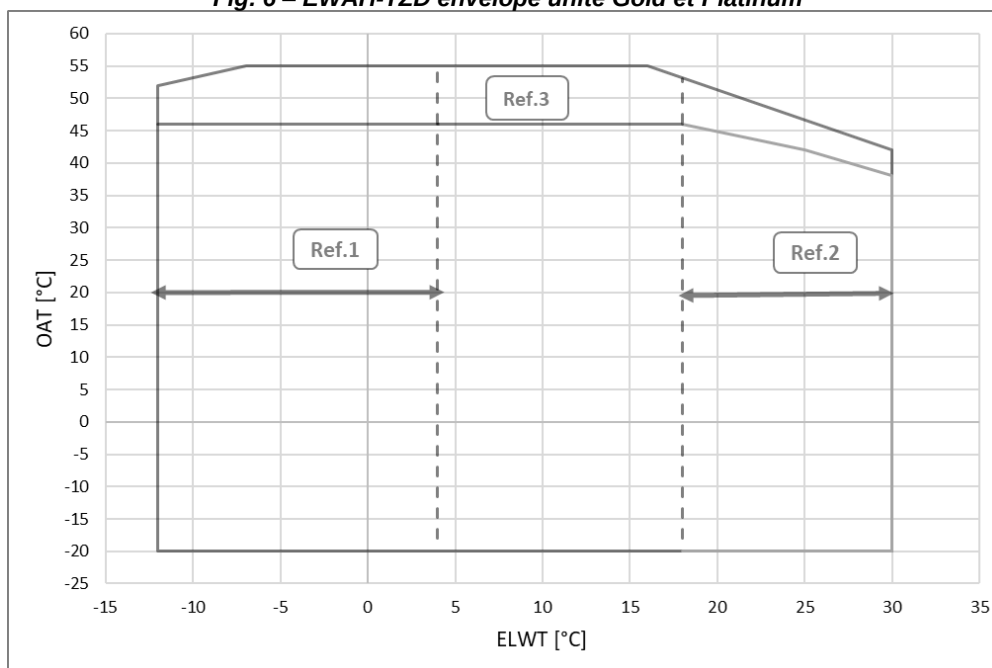
Fig. 6 – EWAH-TZD envelope unité Gold et Platinum
