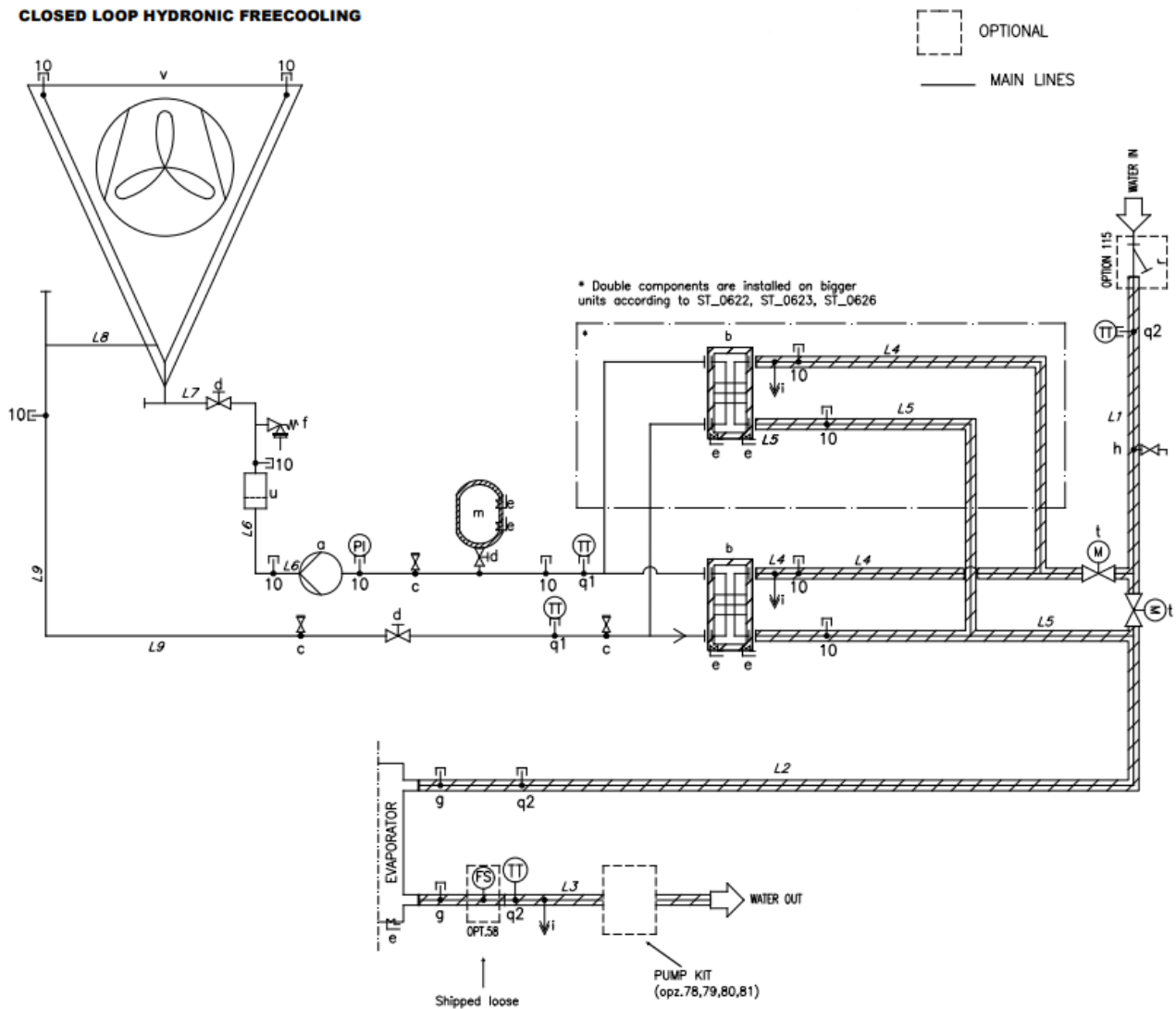
Fig. 29 - P&ID du Free cooling hydronique en boucle fermée (Opt. 231)
