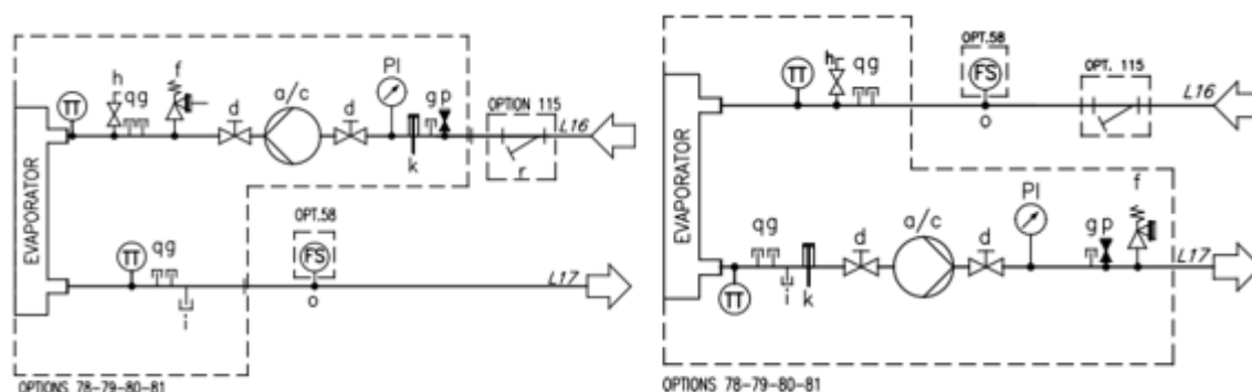
Fig. 27 – Diagramme hydraulique (opt. 78-79-80-81)
