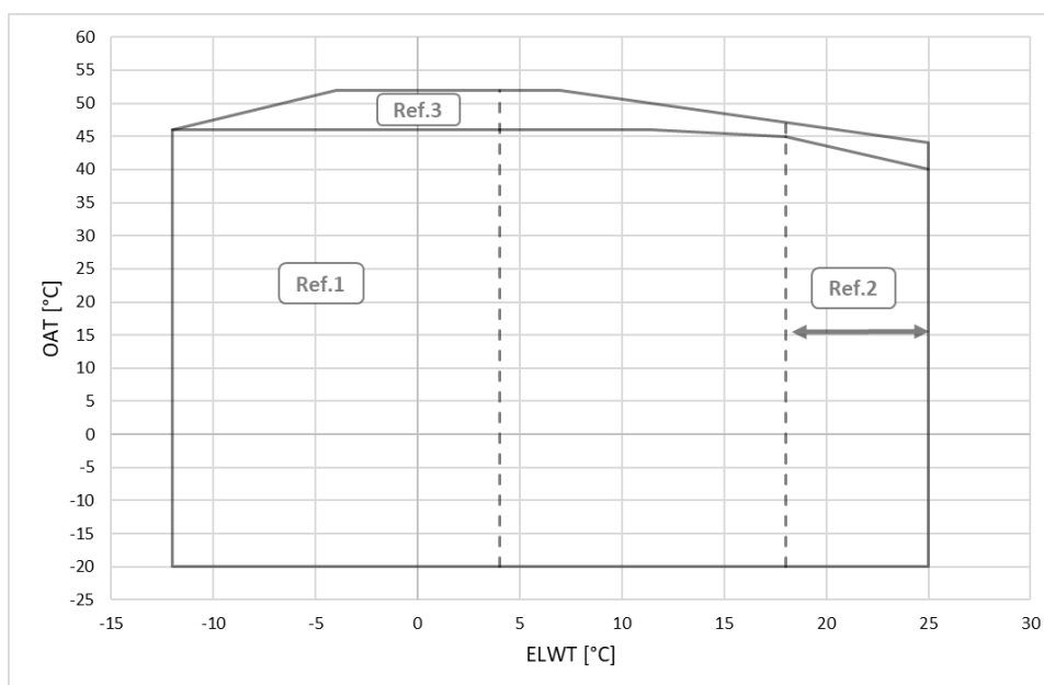
Fig. 16 – EWFD-TZD envelope unité Gold et Platinum
