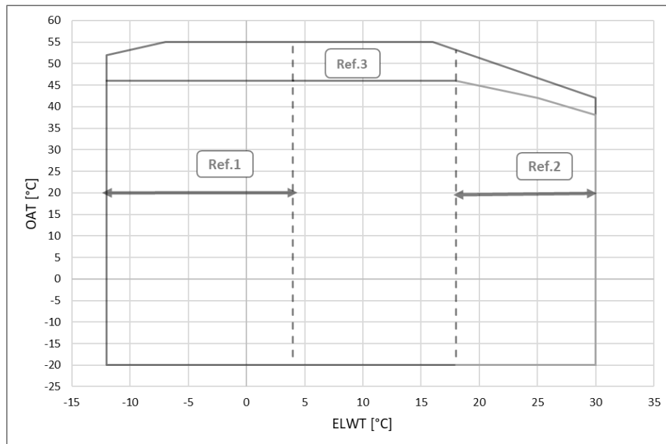
Fig. 14 – EWFH-TZD envelope unité Gold et Platinum
