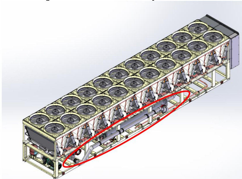
Fig. 30 - Modèles d'unités avec tuyauterie externe
