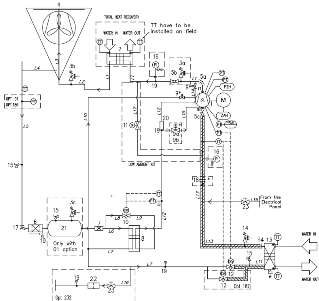
Fig. 1 - Schéma du circuit réfrigérant (P & ID) unité à circuit unique
