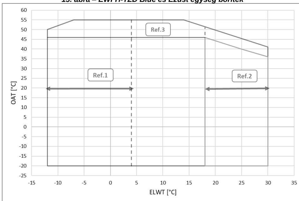
13. ábra – EWFH-TZD Blue és Ezüst egység boríték
