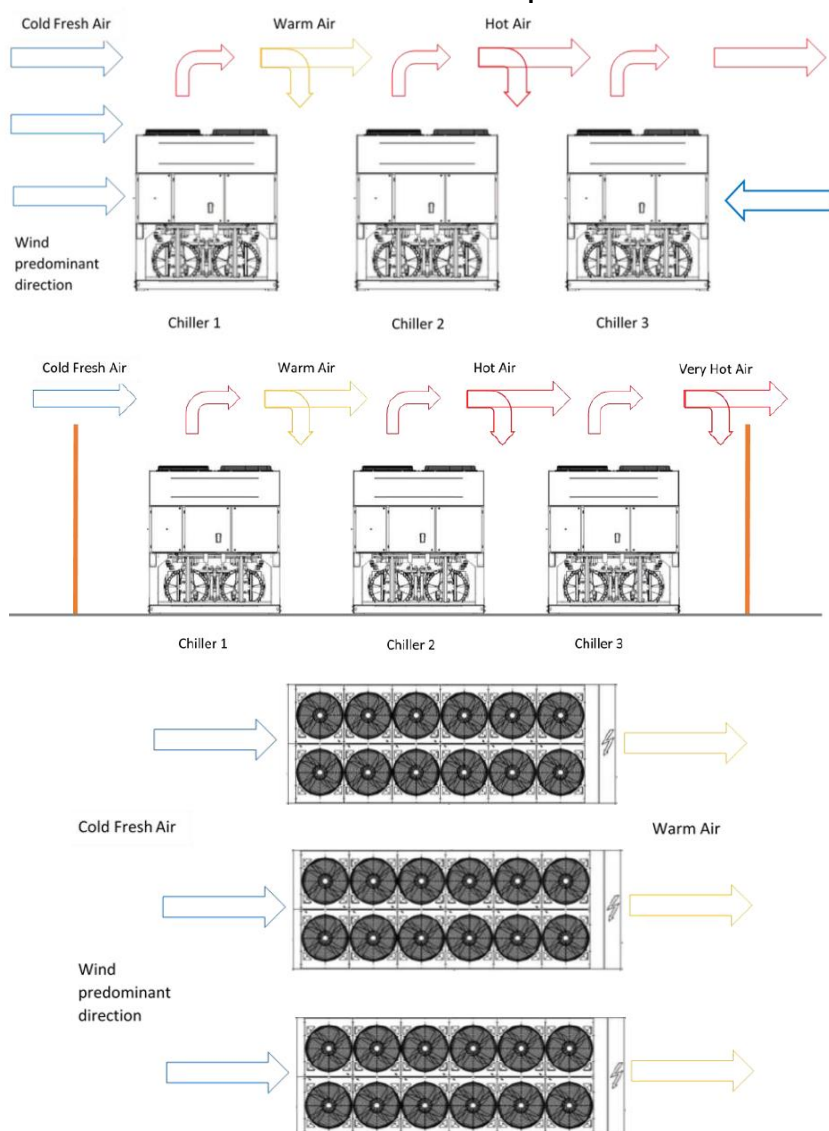
26. ábra – Több hűtő telepítése
