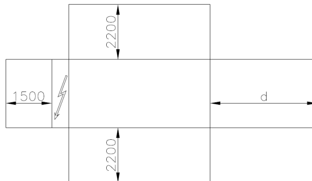
25. ábra - Minimális térszükséglet
