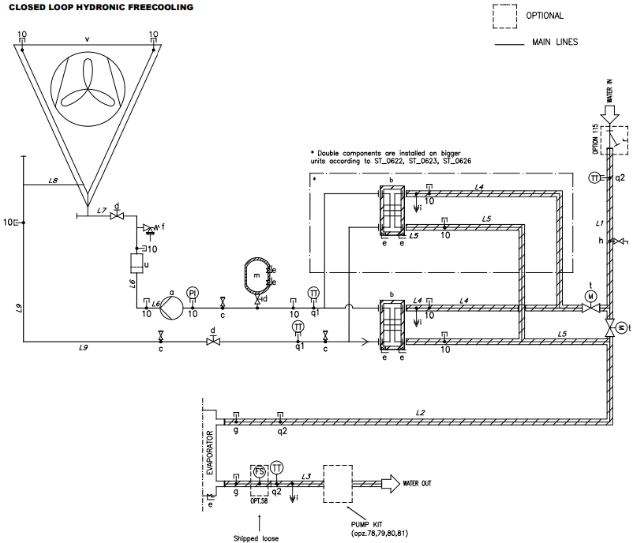
Asztal 1 - Jelmagyarázat Zárt hurok Hidronikus szabad hűtés P&ID
