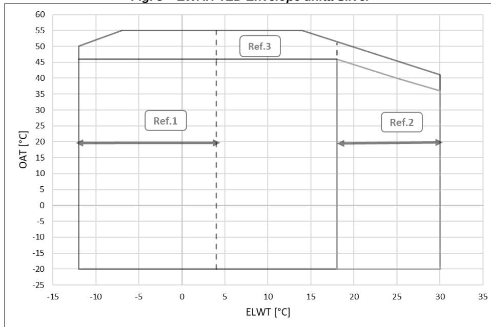
Fig. 5 – EWAH-TZD Envelope unità Silver
