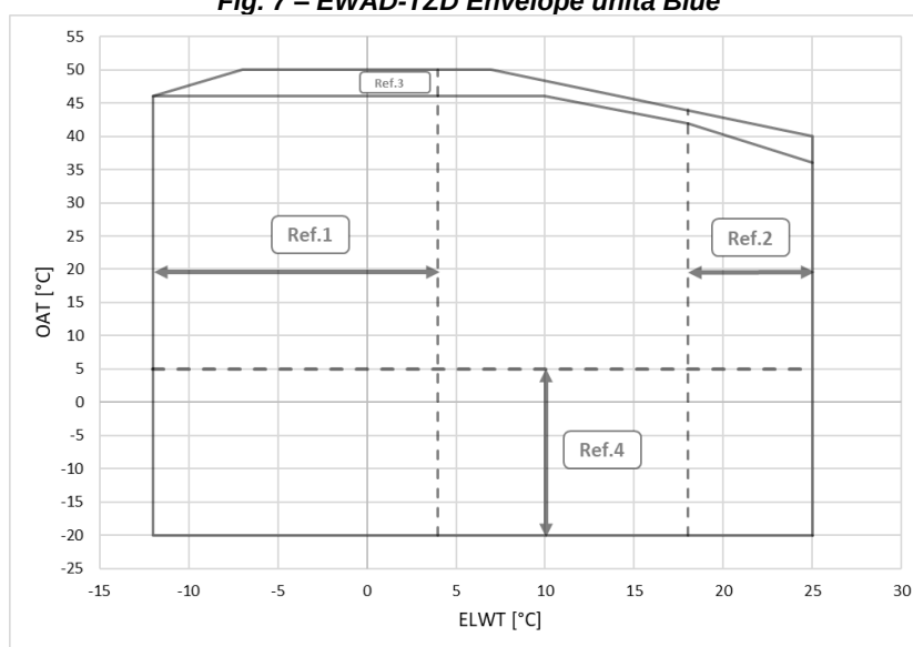
Fig. 7 – EWAD-TZD Envelope unità Blue
