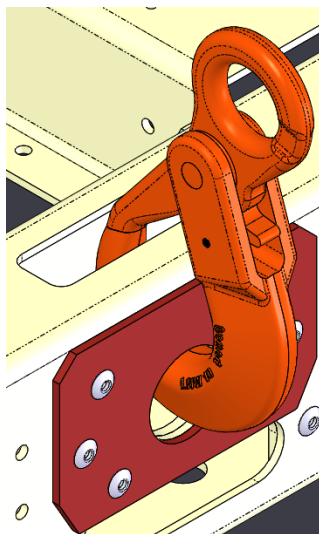
Fig. 19 - Attacco del gancio di sicurezza
