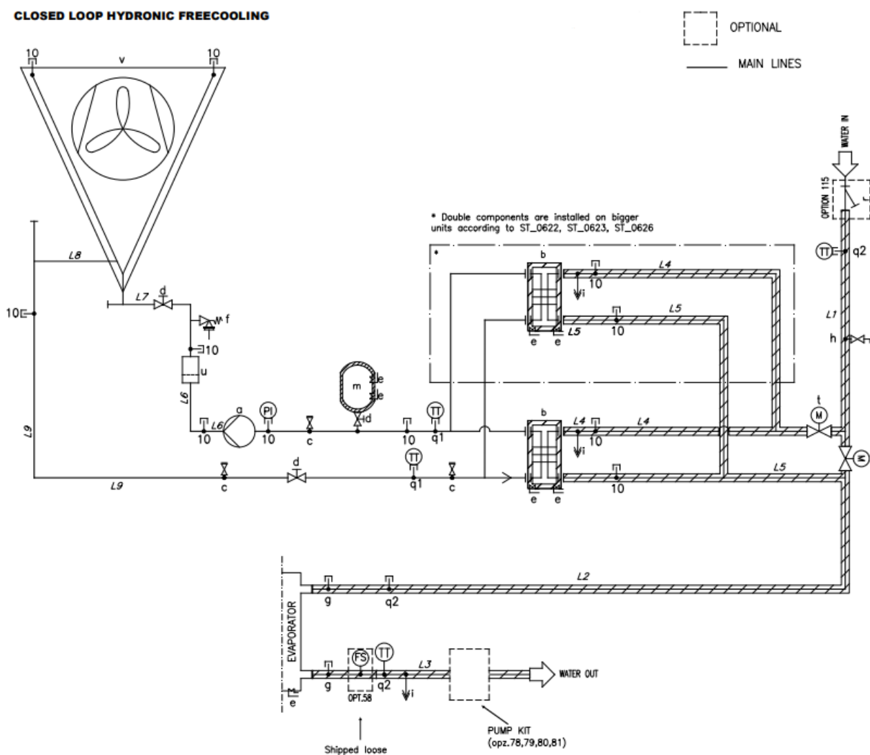
Fig. 29 - P&ID del Free cooling idronico a ciclo chiuso (Opt. 231)
