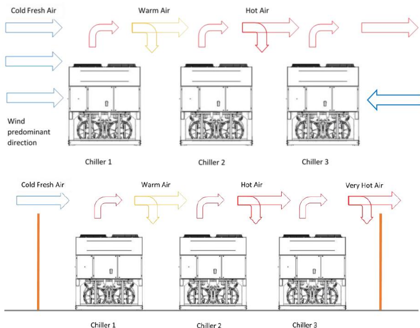
Fig. 26 – Installazione di più chiller
