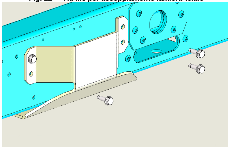
Fig. 22 – Viti M8 per accoppiamento lamiera-telaio
