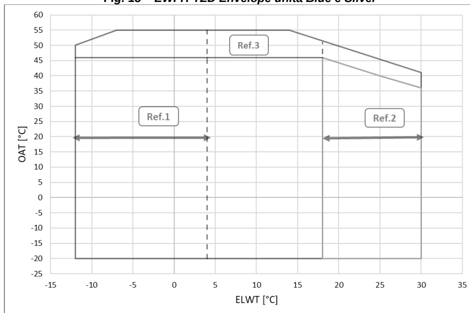
Fig. 13 – EWFH-TZD Envelope unità Blue e Silver
