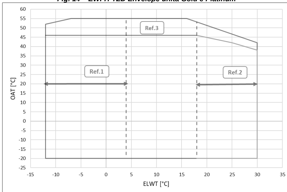
Fig. 14 – EWFH-TZD Envelope unità Gold e Platinum
