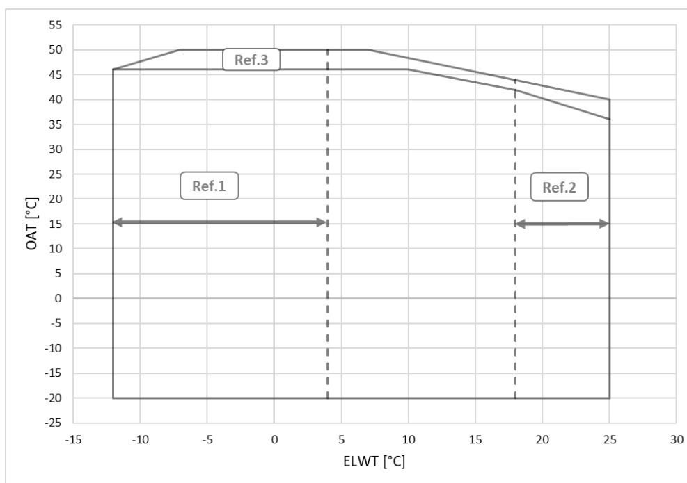
Fig. 15 – EWFD-TZD Envelope unità Blue e Silver
