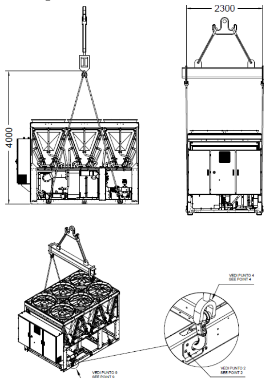
Fig. 18 – Istruzioni di sollevamento
