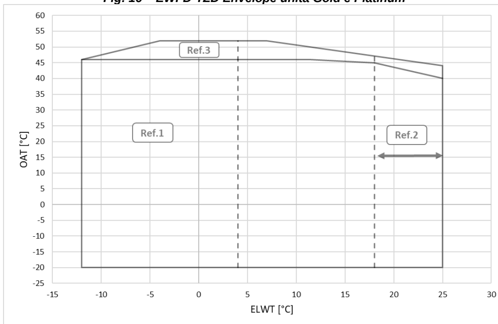
Fig. 16 – EWFD-TZD Envelope unità Gold e Platinum
