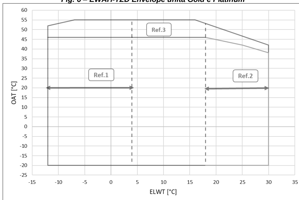
Fig. 6 – EWAH-TZD Envelope unità Gold e Platinum
