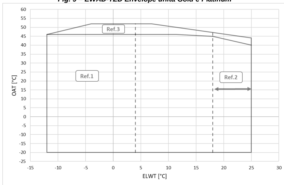
Fig. 9 – EWAD-TZD Envelope unità Gold e Platinum
