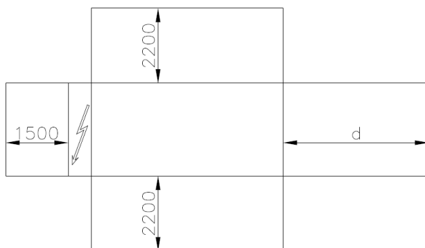
Fig. 25 - Requisiti di spazio minimi
