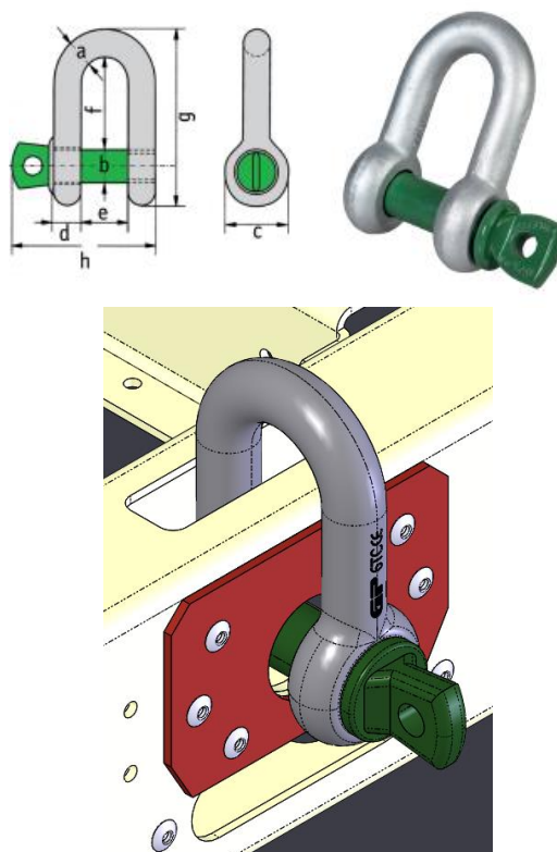
Fig. 20 Fissaggio dei grilli di sollevamento
