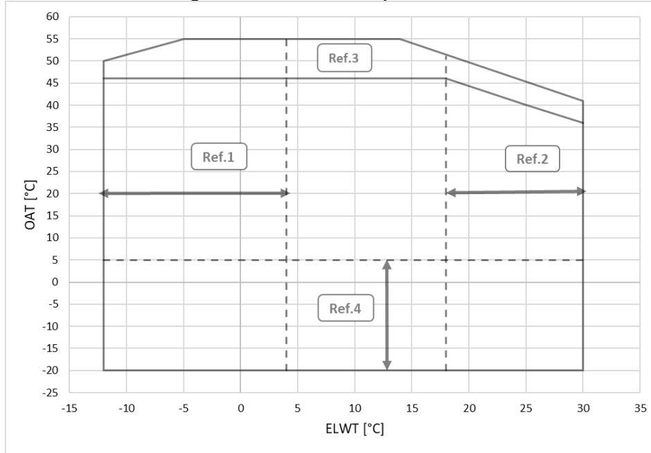
Fig. 5 – EWAH-TZD Envelope unità Silver
