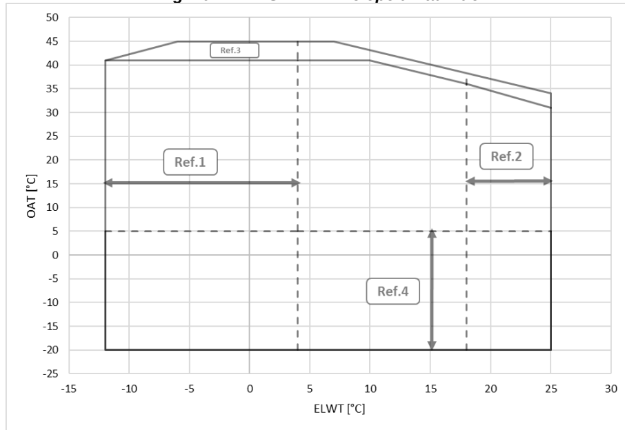
Fig. 11 – EWAS-TZD Envelope unità Silver
