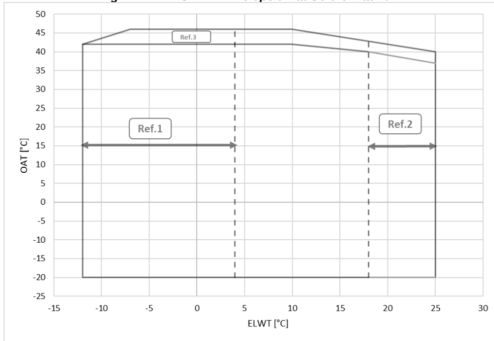
Fig. 12 – EWAS-TZD Envelope unità Gold e Platinum
