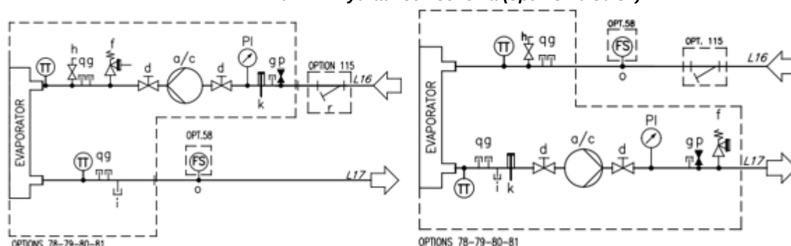
Afb. 27 – Hydraulisch schema (opt. 78-79-80-81)
