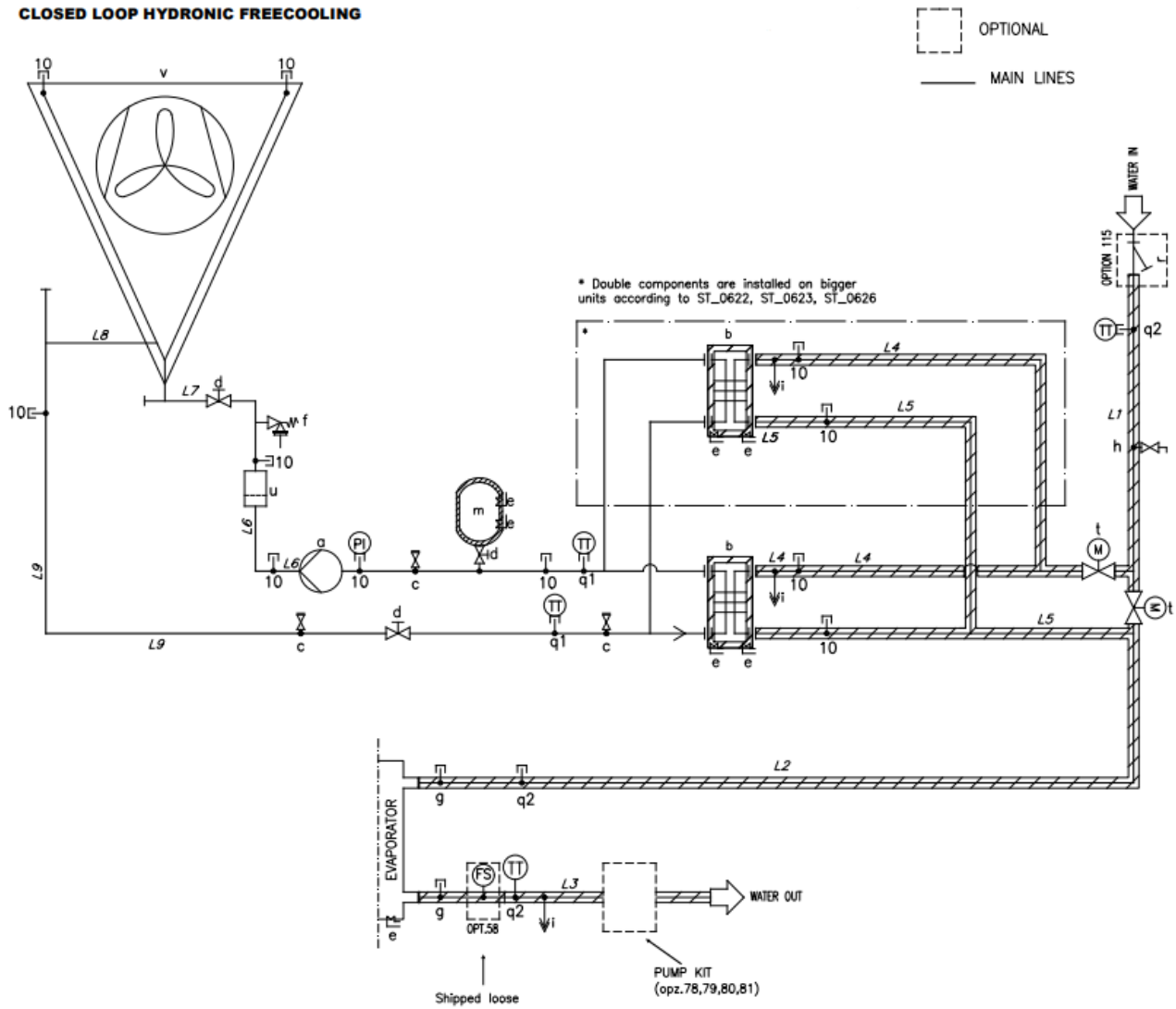
Afb. 29 - Hydronische vrije koeling met gesloten circuit P&ID (Opt. 231)
