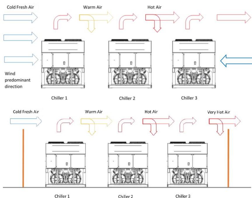
Afb. 26 – Installatie meerdere koelers
