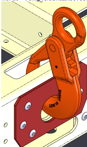
Afb. 19 - Veiligheidshaakbevestiging
