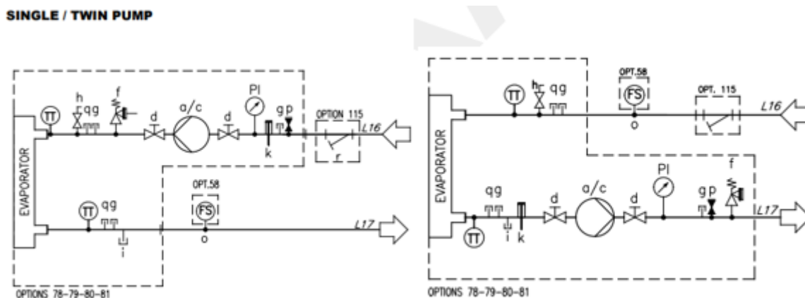
Rys. 27– Schemat hydrauliczny (opt. 78-79-80-81)
