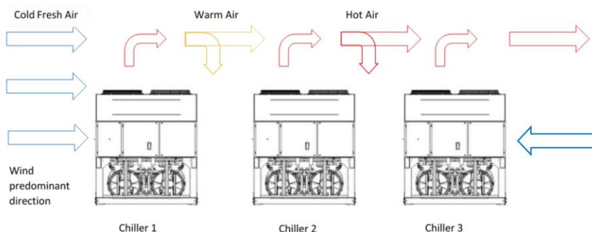
Rys. 26. – Montaż kilku wytwornic wody lodowej
