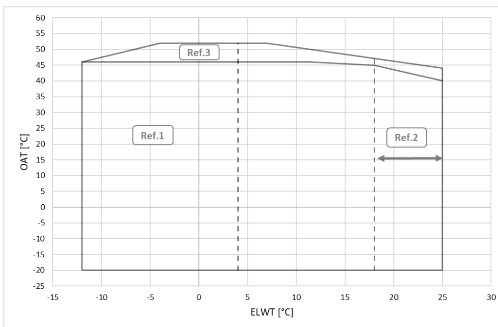
Figura 16– Anvelopa unității EWFD-TZD Gold și Platinum
