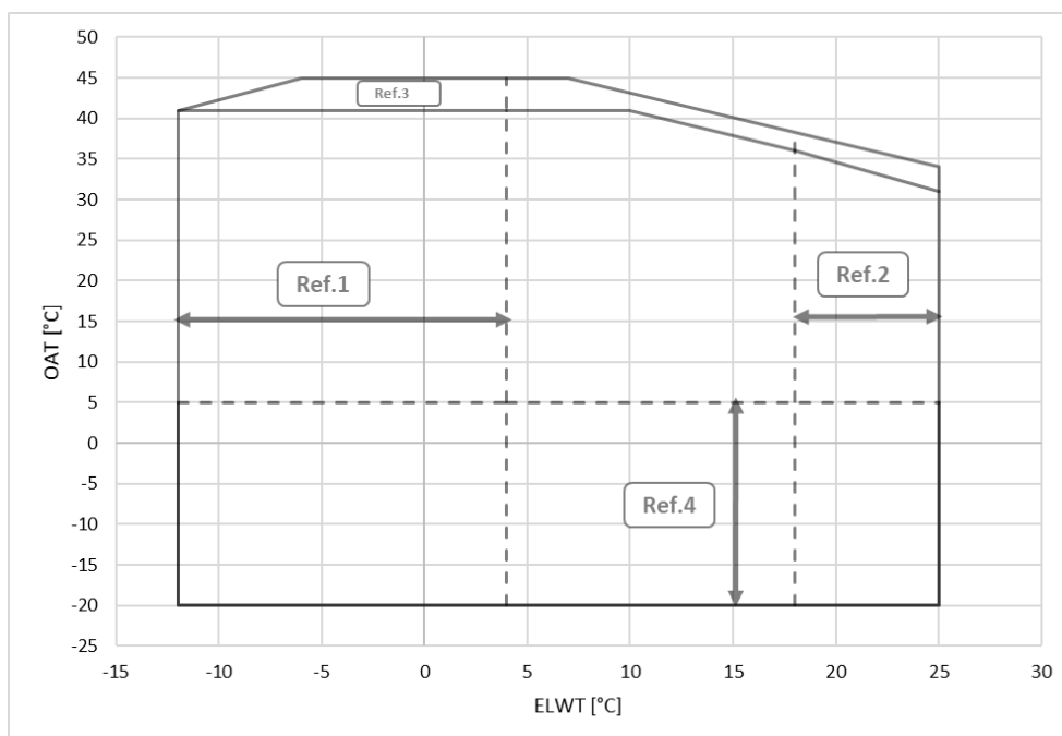
Figura 11– Anvelopă unitate EWAS-TZD Silver
