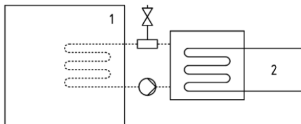
Figura 17- Sistem închis cu ventilație indirectă
