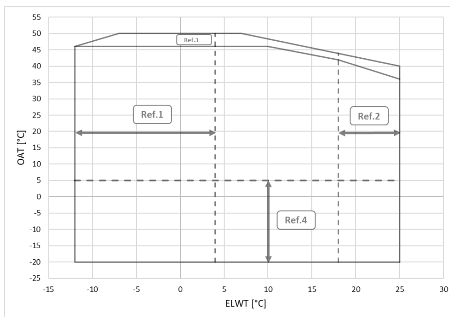
Figura 7– Anvelopă unitate EWAD-TZD Blue
