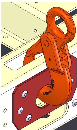
Figura 19- Fixarea cârligului de siguranță
