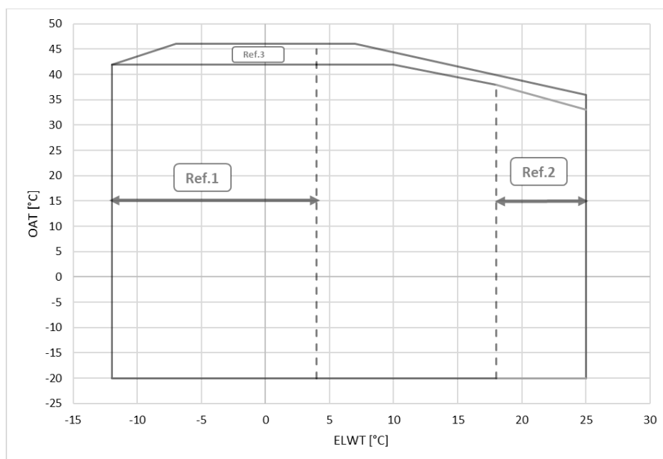
Figura 11– Anvelopă unitate EWAS-TZD Silver
