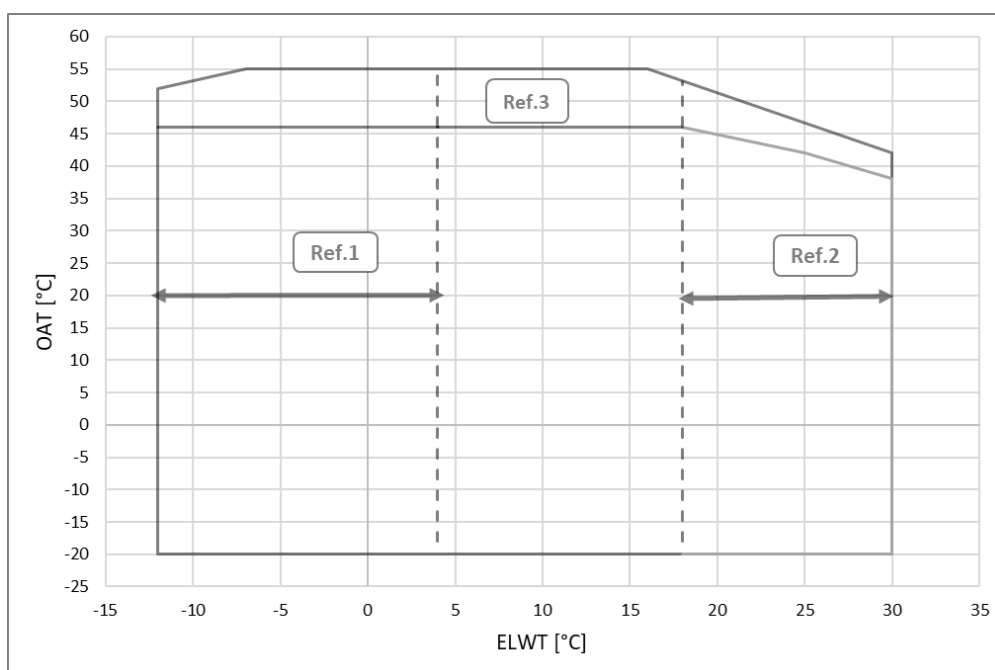
Figura 14– Anvelopă unitate EWFH-TZD Gold și Platinum
