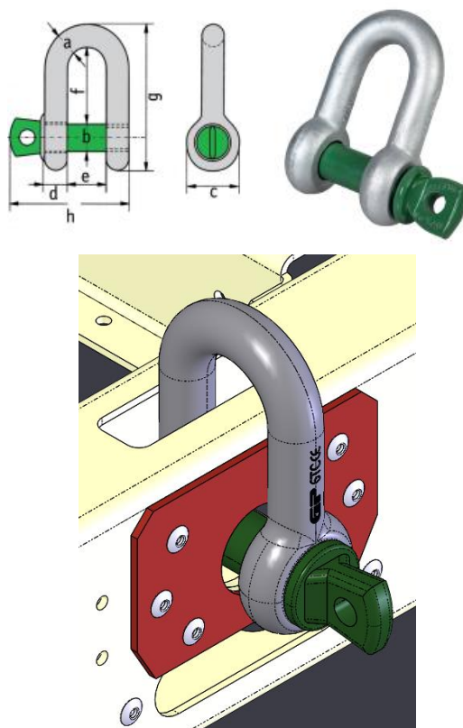
Figura 20 - Fixarea cătușelor de ridicare
