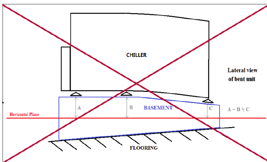
Figura 23– Echilibrarea unității
