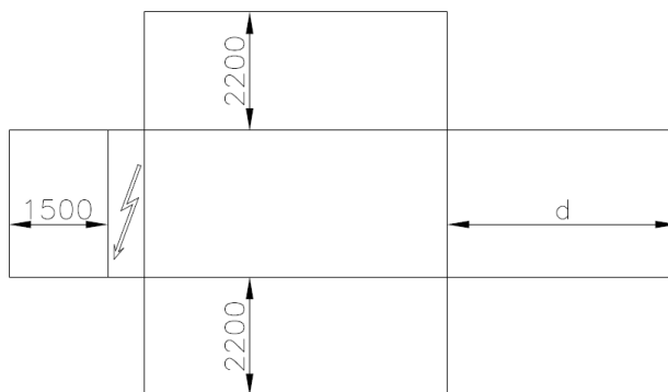
Figura 25- Cerințe minime de spațiu liber
