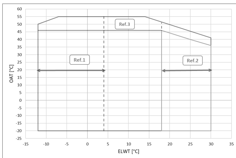
Figura 5– Anvelopă unitate EWAH-TZD Silver
