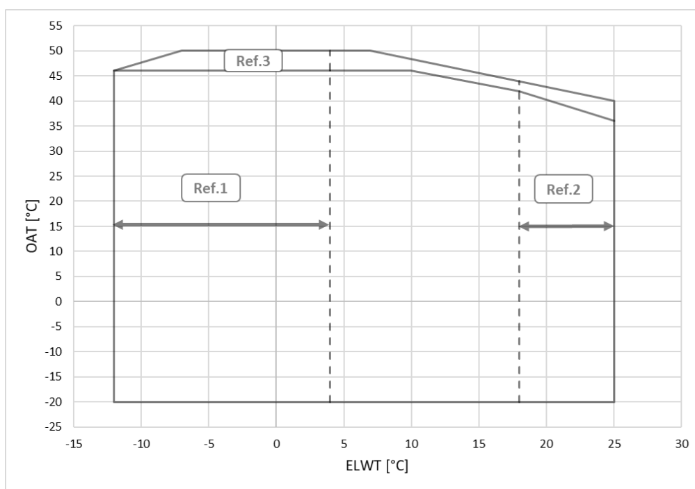
Figura 9– Anvelopă unitate EWAD-TZD Gold și Platinum
