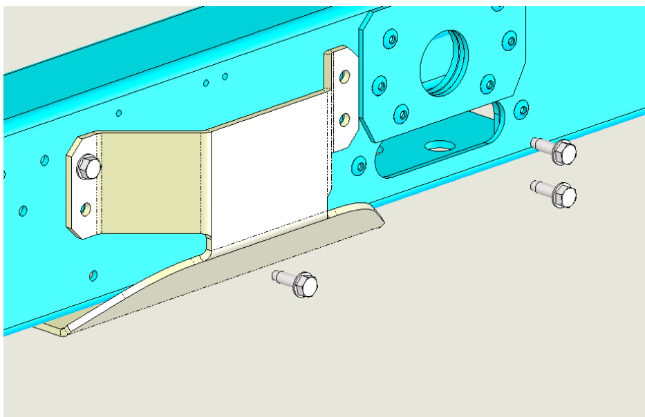
Figura 22 – Șuruburi M8 pentru conectarea cadrului unității la placă
