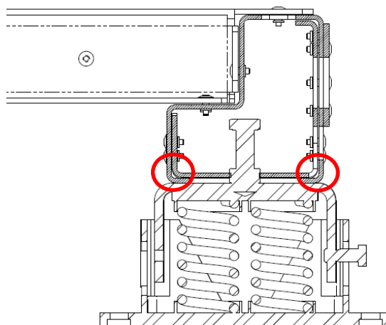
Figura 24– Montarea elementelor anti-vibrații (furnizate opțional)
