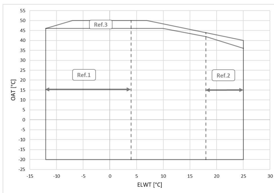
Figura 15– Anvelopa unității EWFD-TZD Blue și Silver
