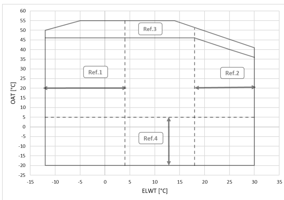
Figura 5– Anvelopă unitate EWAH-TZD Silver
