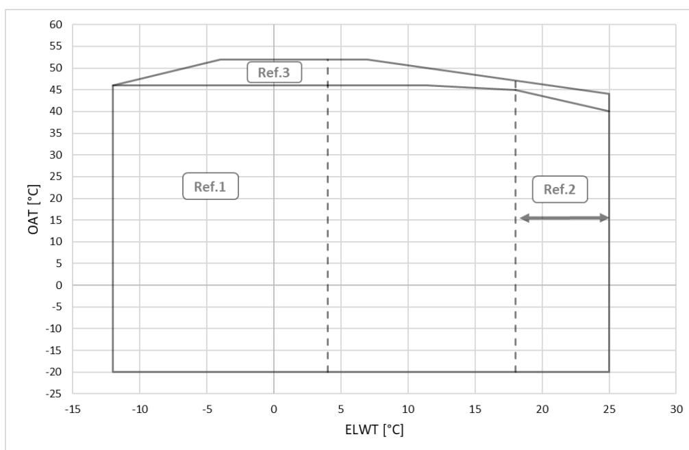
Figura 9– Anvelopă unitate EWAD-TZD Gold și Platinum
