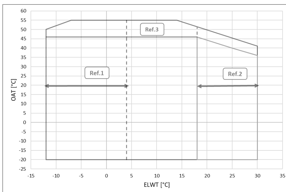
Figura 13– Anvelopă unitate EWFH-TZD Blue și Silver
