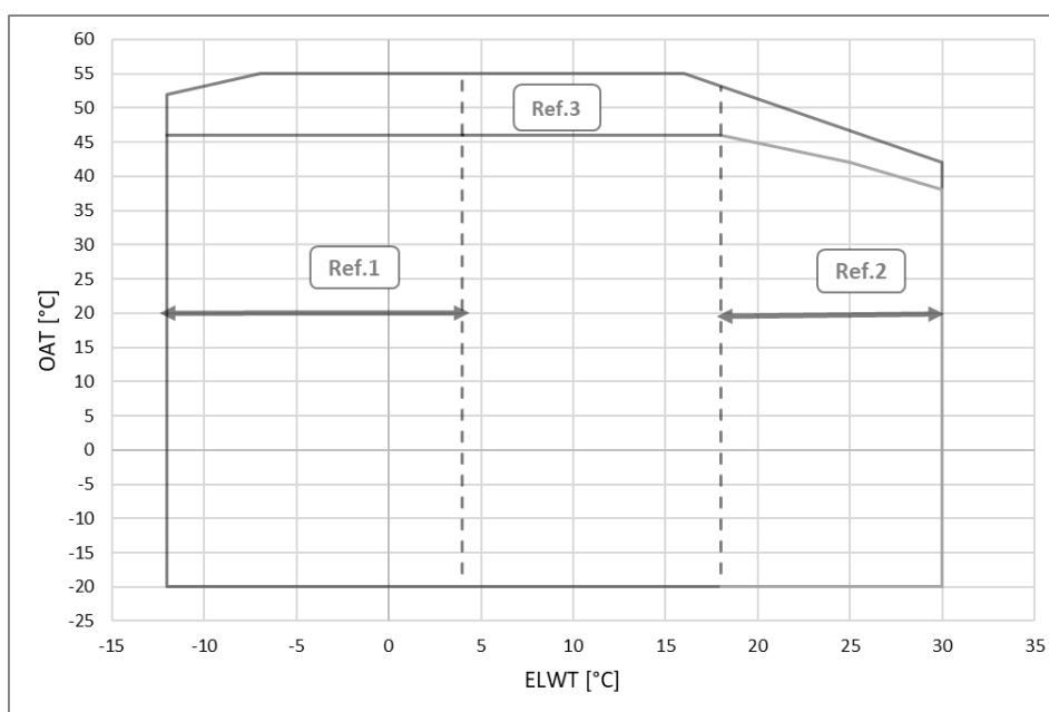
Figura 6– Anvelopă unitate EWAH-TZD Gold și Platinum
