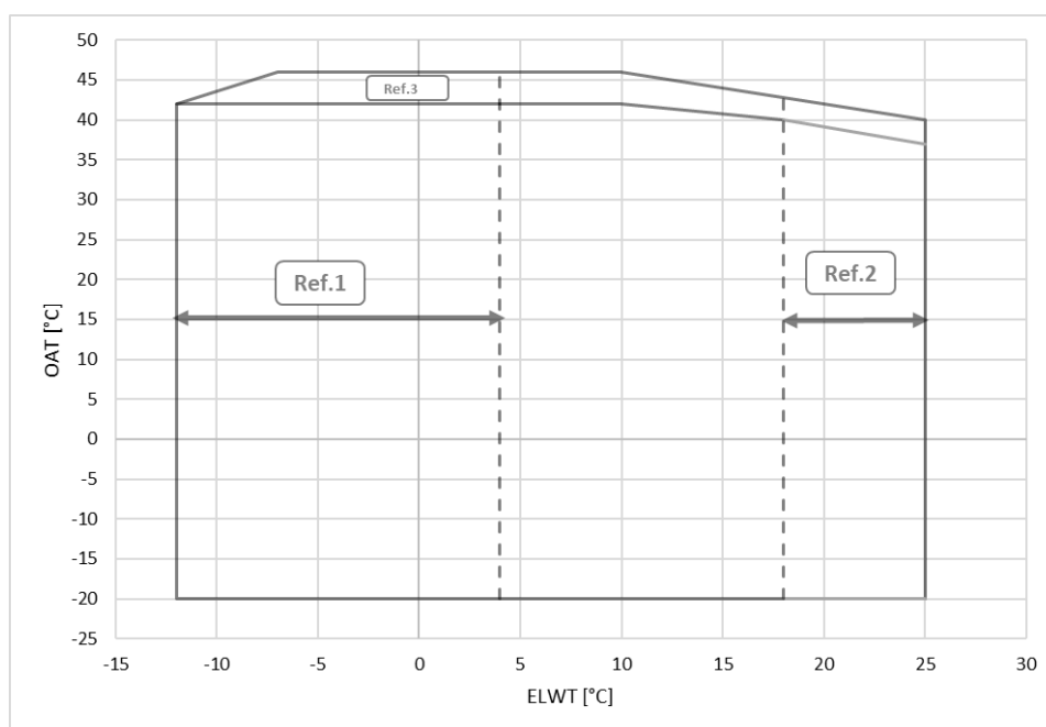
Figura 12– Anvelopă unitate EWAS-TZD Gold și Platinum
