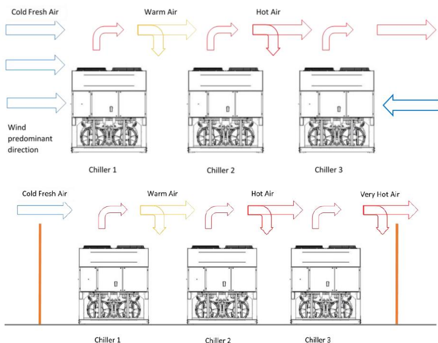
Figura 26. – Instalarea mai multor dispozitive de răcire
