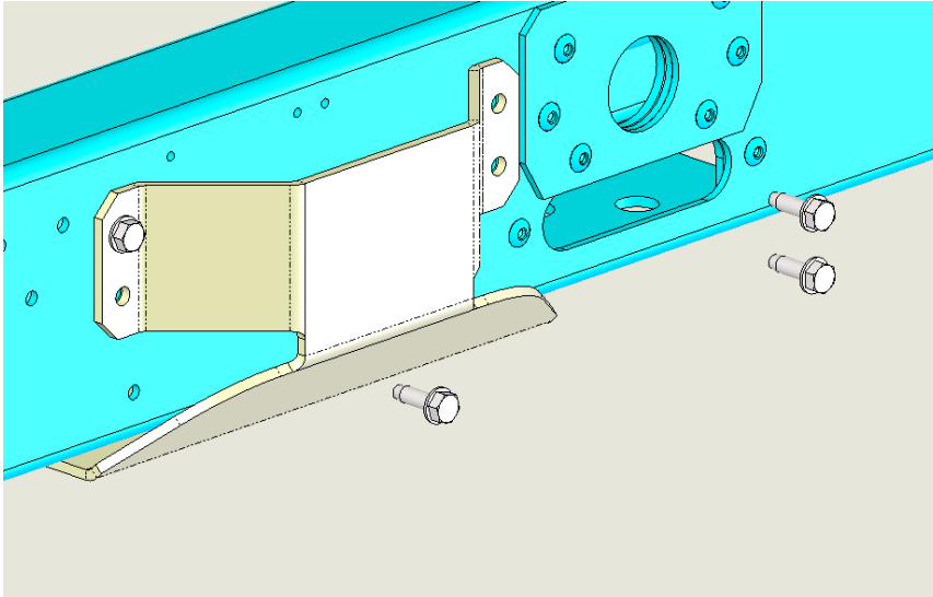
Şek. 22 – Plaka-ünite çerçeve bağlantısı için M8 cıvataları
