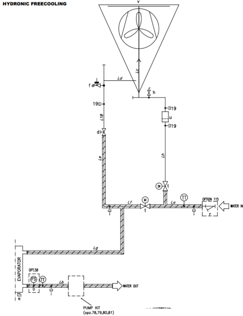
Şek. 28- Hidronik Serbest Soğutma P&ID
