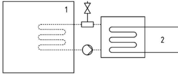
Şekil 17- Dolaylı havalandırılmalı kapalı sistem
