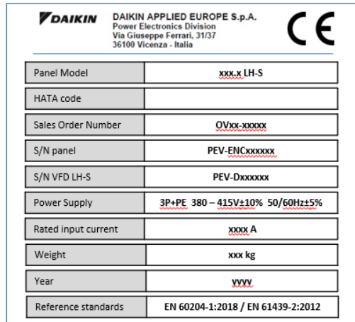
Şek. 32- Elektrik Panosu Tanımlama Etiketi
