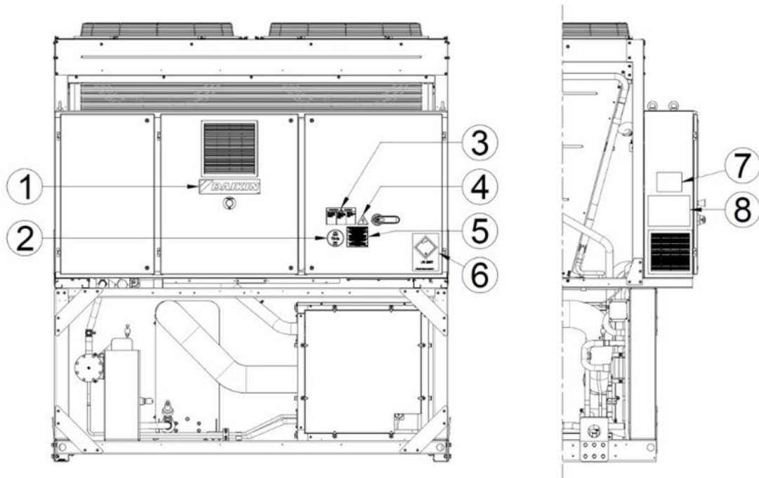
Fig. 4 – Descrizione delle etichette applicate sul pannello elettrico
