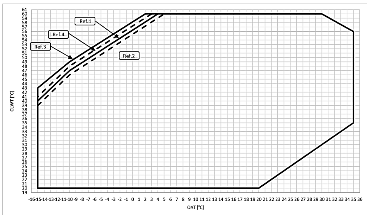
Фиг.° 7 - EWYT-B-S - OP.204 Работни граници в режим на отопление
