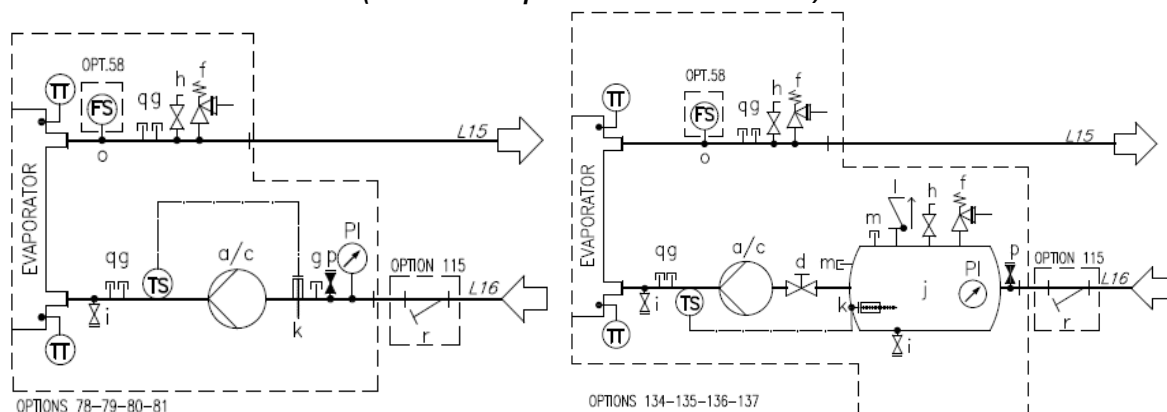
Фиг. ° 17 - Хидравлична схема за двойна помпа (EWYTx5B) (опт. 80-81/136-137) (максимално работно налягане 6 bar)
