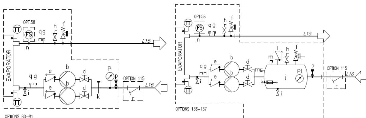
Фиг. ° 17 - Хидравлична схема за двойна помпа (EWYTx5B) (опт. 80-81/136-137) (максимално работно налягане 6 bar)
