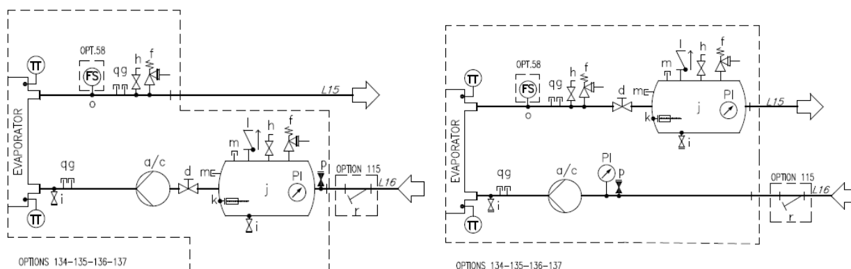
Фиг.° 16 - Хидравлична схема за единична помпа/двойна помпа с резервоар (EWYTx5B) (опт. 134-135) (максимално работно налягане 6 bar)
