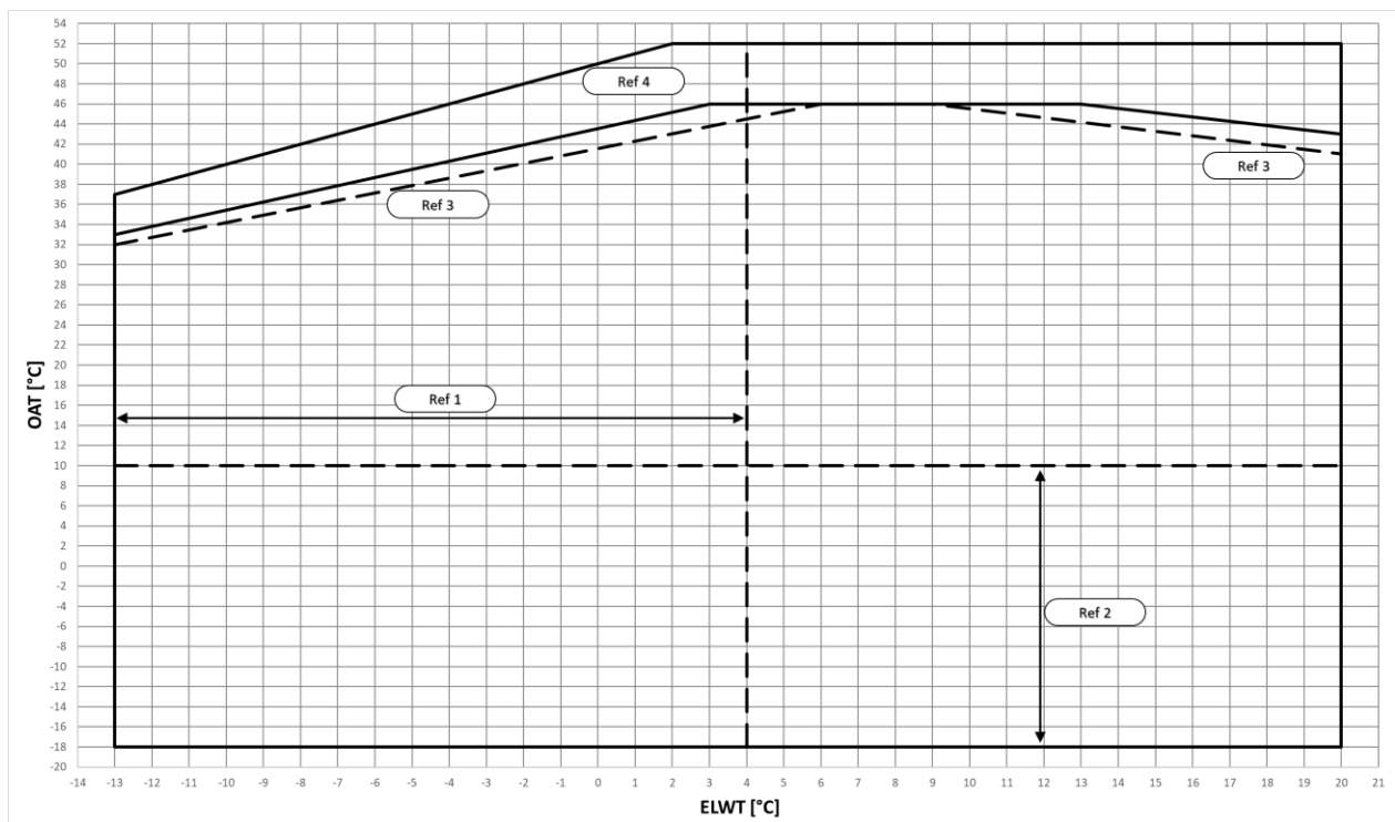
Abb. 3 – EWYTx0B-S Betriebsgrenzen im Kühlbetrieb
