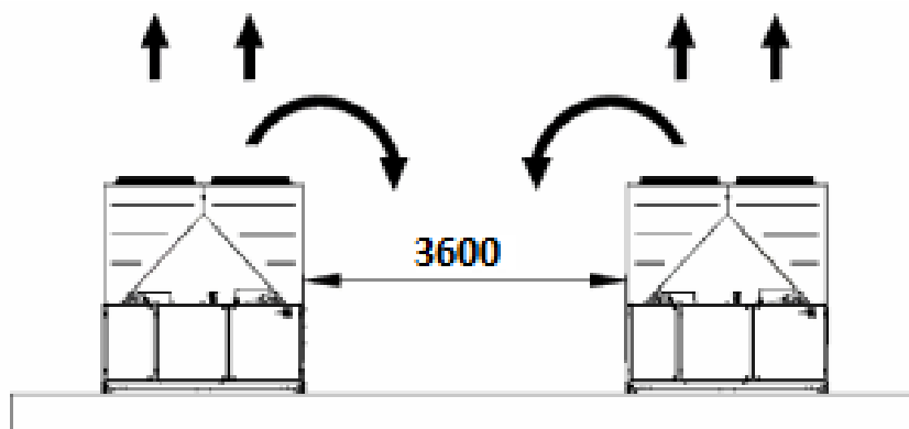
Abb. 11 – Mindestabstände
