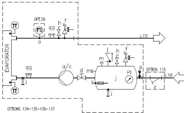
Εικ. 16 – Διάγραμμα υδραυλικού κυκλώματος για μονή αντλία / διπλή αντλία με δεξαμενή (EWYTx5B) (επιλογές 134-135) (μέγιστη πίεση λειτουργίας 6 bar)
