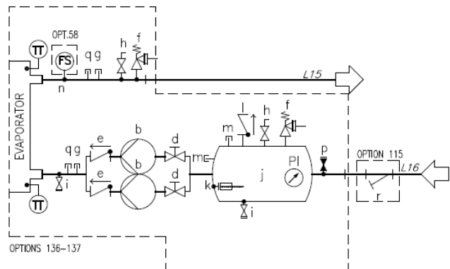
Εικ. 17 – Διάγραμμα υδραυλικού κυκλώματος για διπλή αντλία (EWYTx5B) (επιλογές 80-81/136-137) (μέγιστη πίεση λειτουργίας 6 bar)
