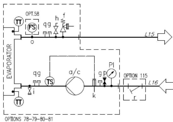
Εικ. 18 – Διάγραμμα υδραυλικού κυκλώματος για μονή αντλία / διπλή αντλία (επιλογές 78-79-80-81/134-135-136-137) (μέγιστη πίεση λειτουργίας 6 bar)
