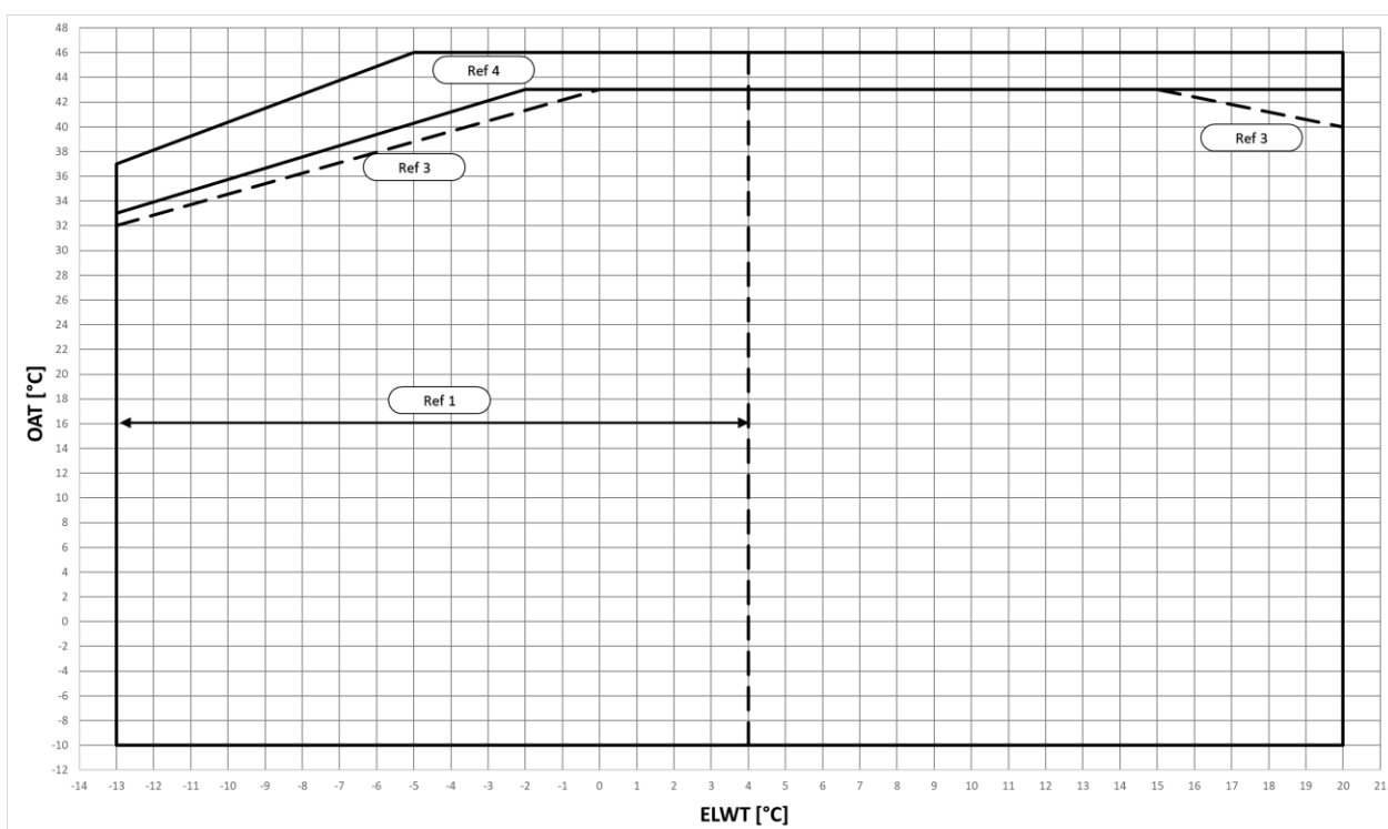
Εικ. 1 – Όρια λειτουργίας ψύξης μονάδας EWYTx5B-S
