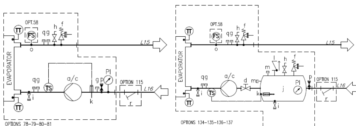
Fig. 18 - Schéma hydraulique pour pompe unique/pompes jumelles (opt. 78-79-80-81/134-135-136-137) (pression de service max. 6 bar)
