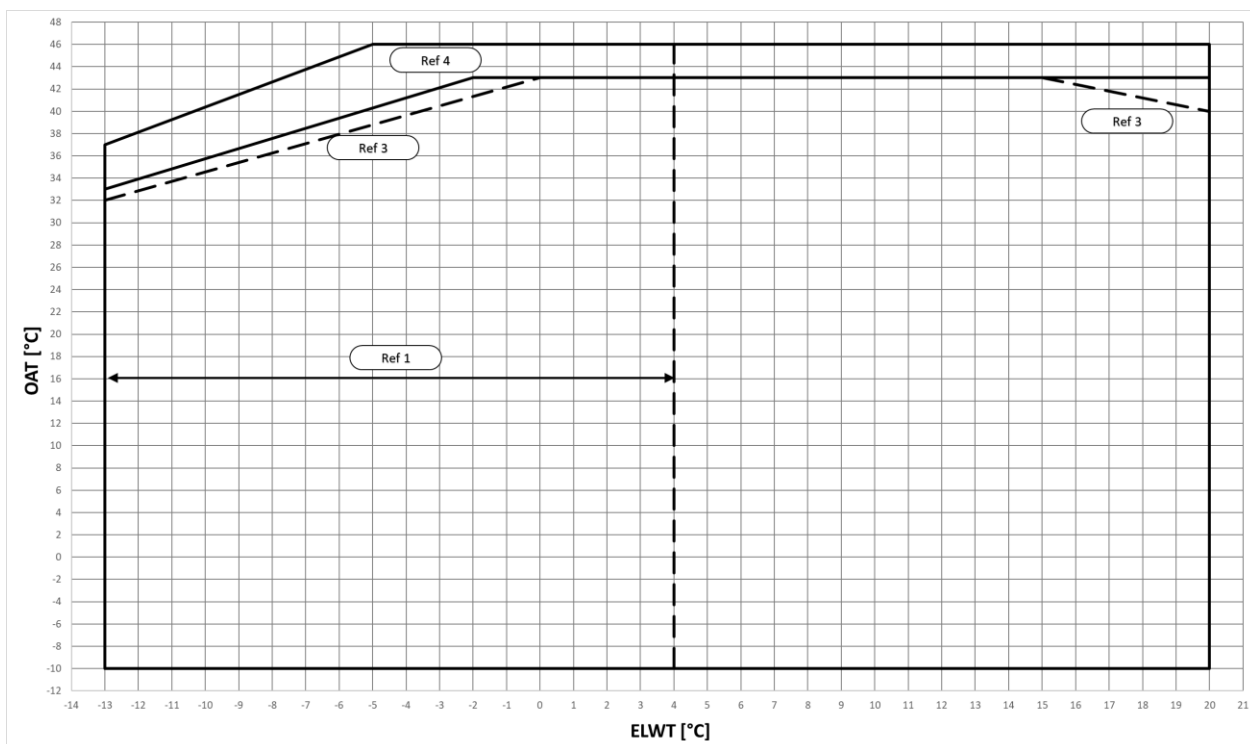
1. ábra – EWYTx5B-S üzemeltetési határértékei hűtés módban
