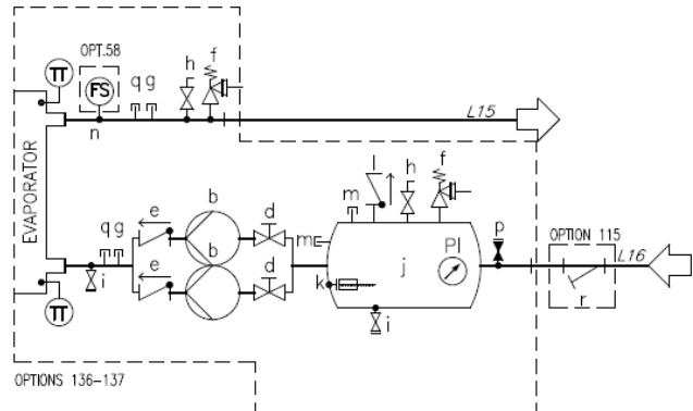
17. ábra – Dupla szivattyú hidraulikus diagramja (EWYTx5B) (opt. 80-81/136-137) (max. üzemi nyomás 6 bar)
