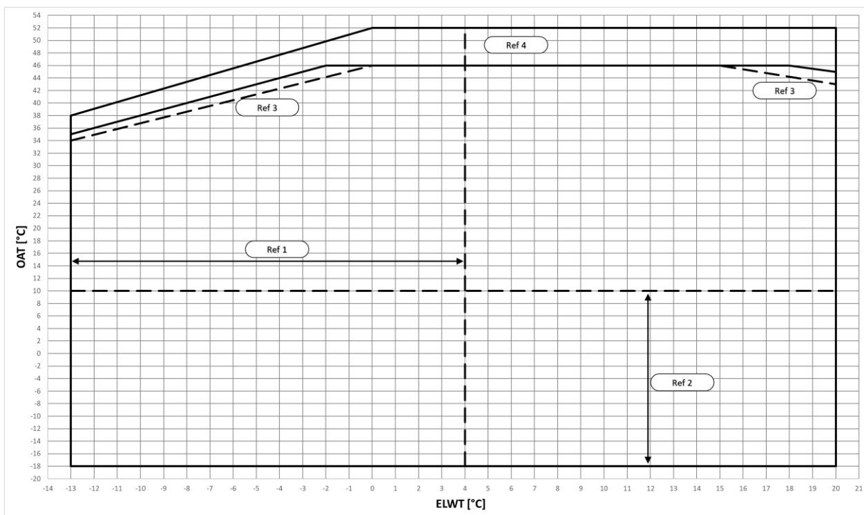
4 . ábra – EWYTx0B-X üzemeltetési határértékei hűtés módban
