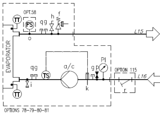
18. ábra – Hidraulikus diagram egy szivattyúhoz / ikerszivattyúhoz (opt. 78-79-80-81/134-135-136-137) (max. üzemi nyomás 6 bar)
