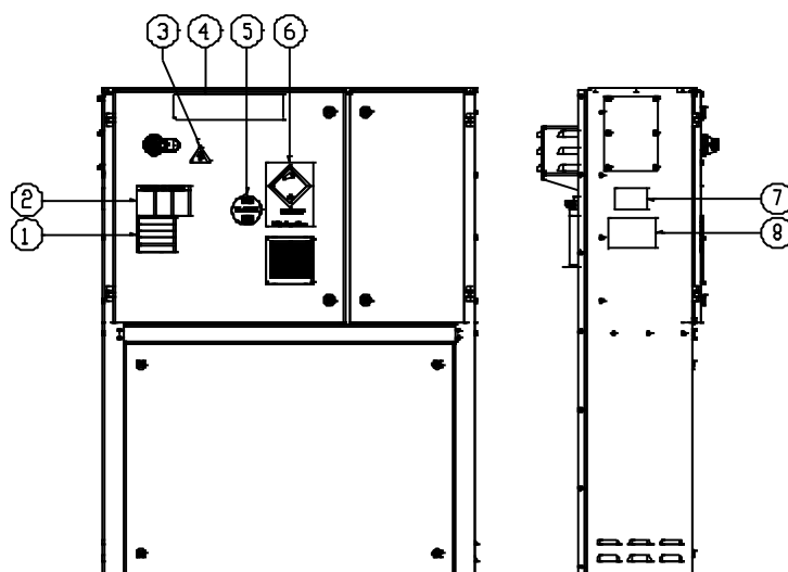
22. ábra - Az elektromos burkolatokon elhelyezett címkék értelmezése EWYTxx5B
