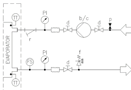
14 pav. – Hidraulikos schema be įrengto siurblio (-ių) (maks. darbinis slėgis 20 barų)
