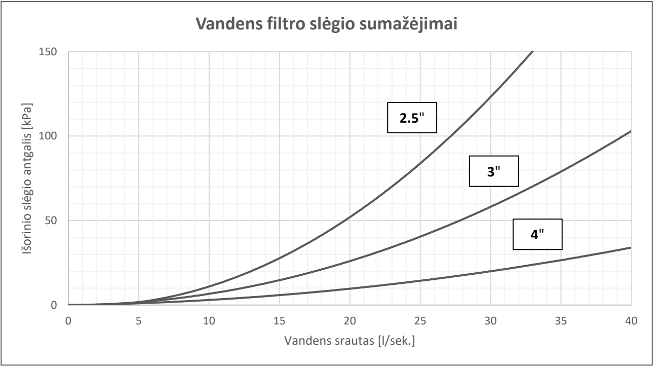
13 pav. – Vandens filtro slėgio sumažėjimas
