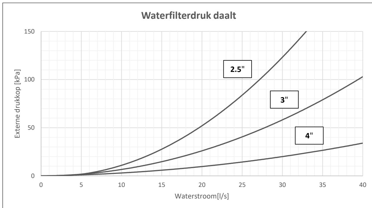
Afb. 13 – Drukvermindering waterfilter
