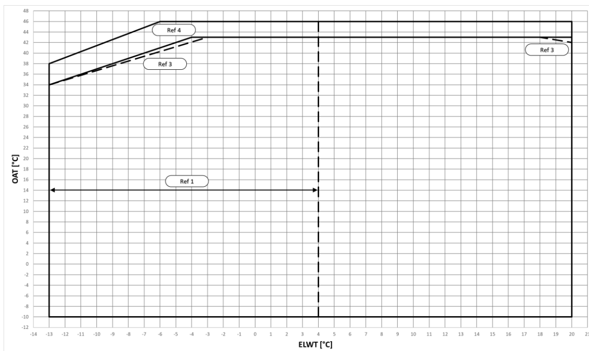
Afb. 2 – EWYTxx5B-X Operationele limieten modus koeling
