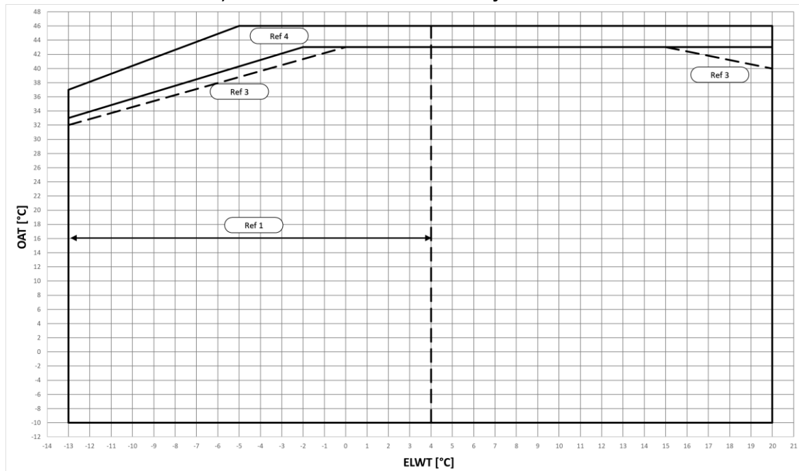
Afb. 1 – EWYTxx5B-S Operationele limieten modus koeling
