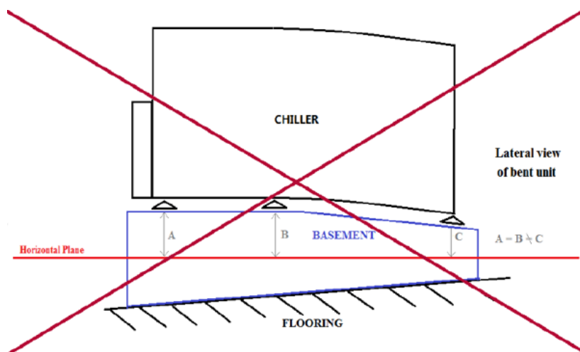
Afb. 10 – Nivelleringsysteem
