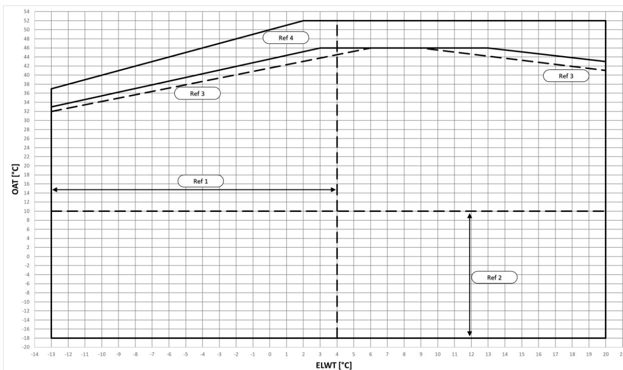
Afb. 3 – EWYTxx0B-S Operationele limieten modus koeling
