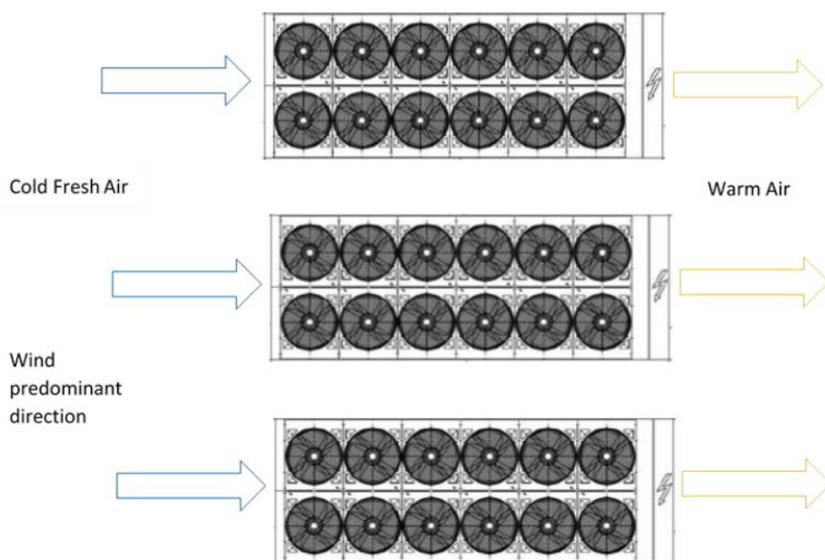
Afb. 12 – Installatie meerdere systemen (modus koeling)
