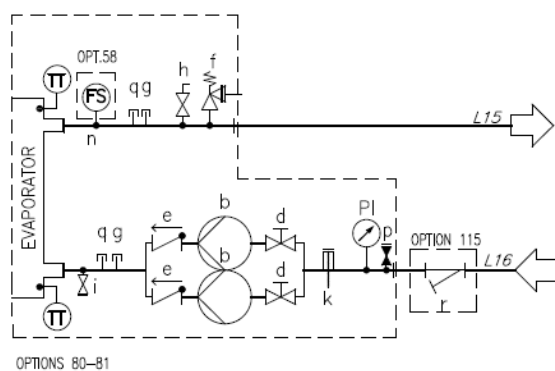
Rys. 17 — Schemat hydrauliczny pompy podwójnej (EWYTx5B) (opcja 80-81/136-137) (maks. ciśnienie robocze 6 bar)
