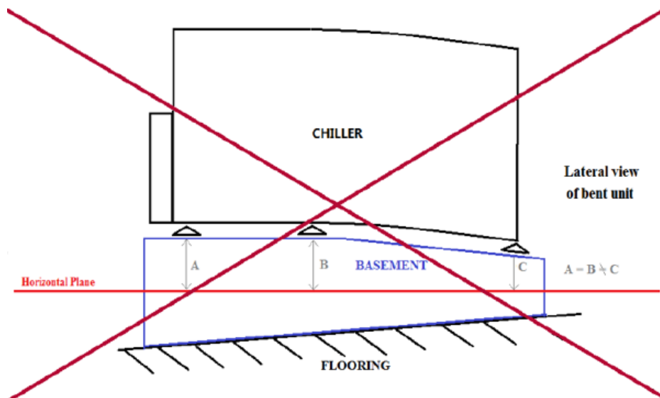
Rys. 10 — Poziomowanie jednostki
