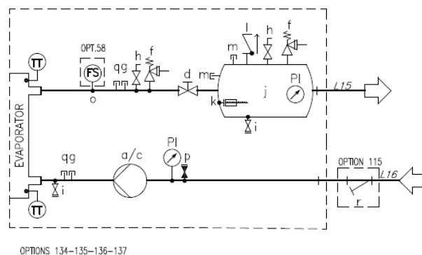
Rys. 16 — Schemat hydrauliczny pompy pojedynczej/pompy podwójnej ze zbiornikiem (EWYTx5B) (opcja 134-135) (maks. ciśnienie robocze 6 bar)
