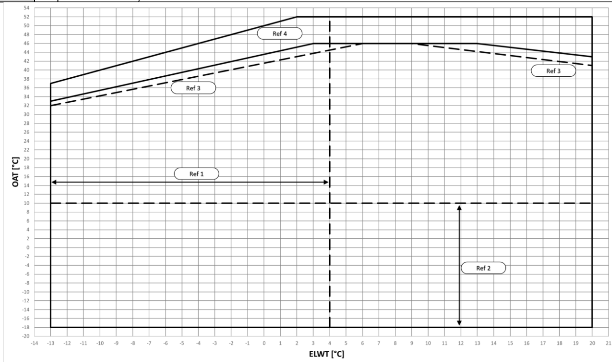
Rys. 3 — EWTxx0B-S — limity operacyjne trybu chłodzenia
