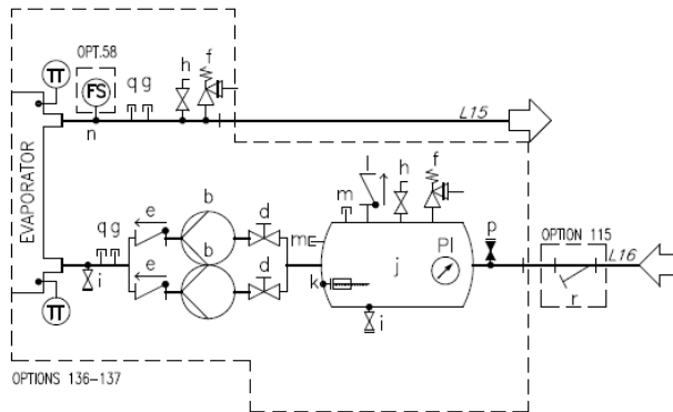
Rys. 17 — Schemat hydrauliczny pompy podwójnej (EWYTx5B) (opcja 80-81/136-137) (maks. ciśnienie robocze 6 bar)
