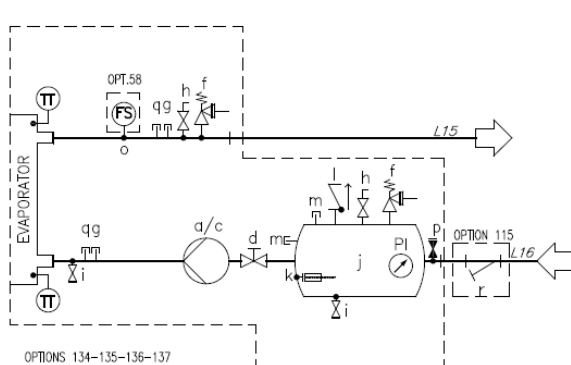
Rys. 16 — Schemat hydrauliczny pompy pojedynczej/pompy podwójnej ze zbiornikiem (EWYTx5B) (opcja 134-135) (maks. ciśnienie robocze 6 bar)
