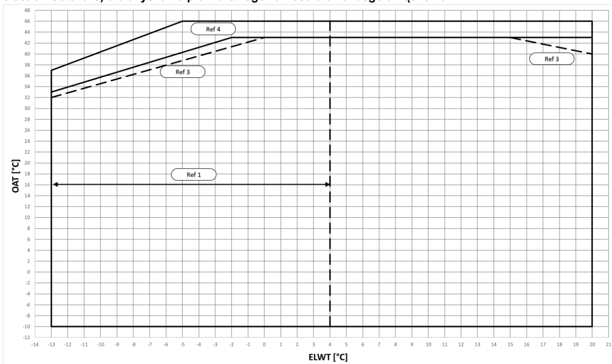
Rys. 1 — EWYTxx5B-S — limity operacyjne trybu chłodzenia
