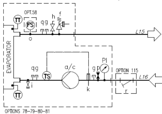
Rys. 18 — Schemat hydrauliczny pompy pojedynczej/pompy podwójnej (opcja 78-79-80-81/134-135-136-137) (maks. ciśnienie robocze 6 bar)
