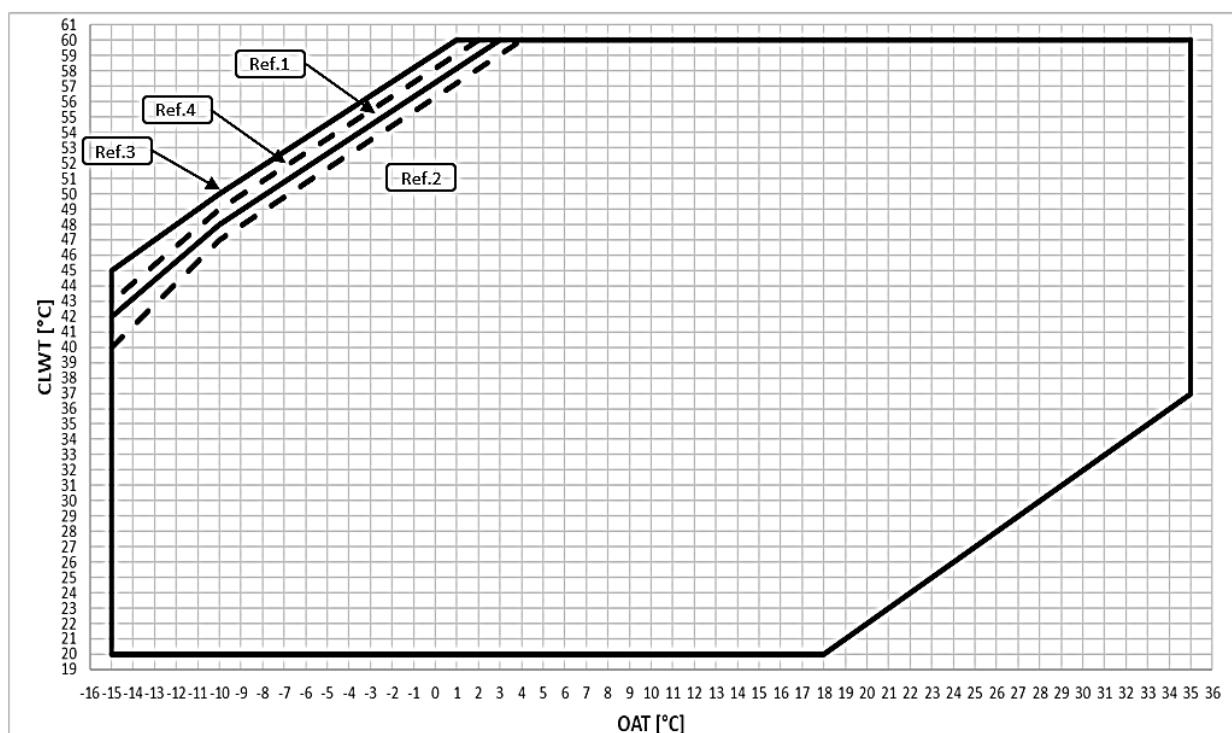
Rys. 8 — EWT~B-X — limity operacyjne trybu ogrzewania OP.204
