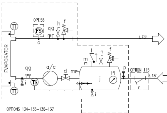
Rys. 18 — Schemat hydrauliczny pompy pojedynczej/pompy podwójnej (opcja 78-79-80-81/134-135-136-137) (maks. ciśnienie robocze 6 bar)
