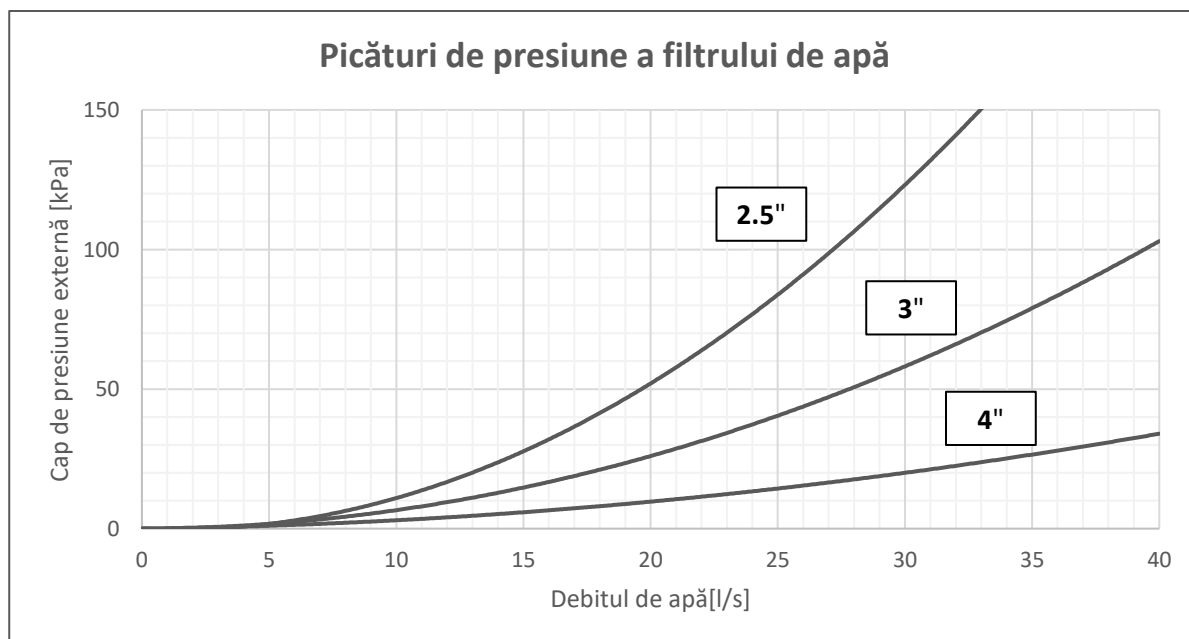
Fig. 13 –Cădere de presiune a filtrului de apă
