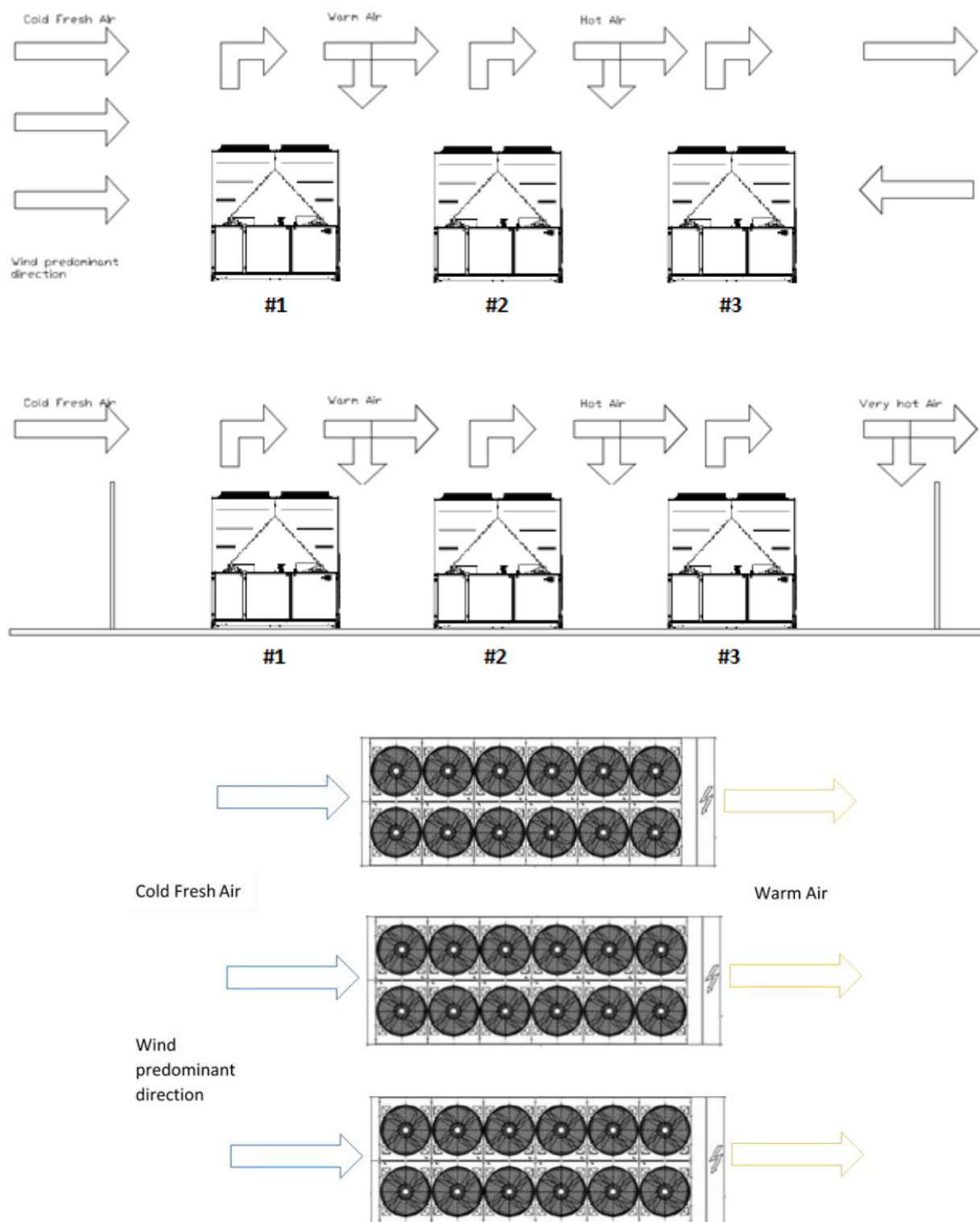
Fig. 12 – Instalarea mai multor răcitoare
