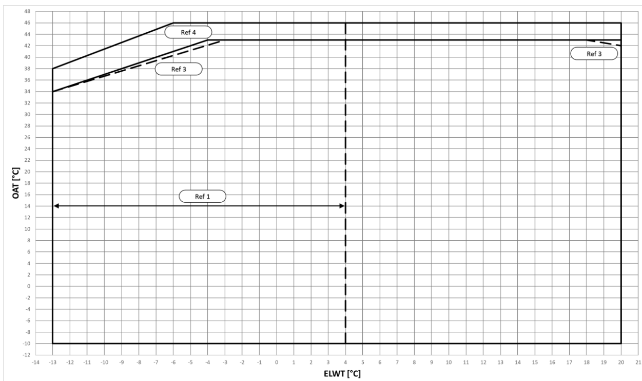
Fig. 2 – EWYTx5B-X Limitele Operationale ale Modulului de Racire
