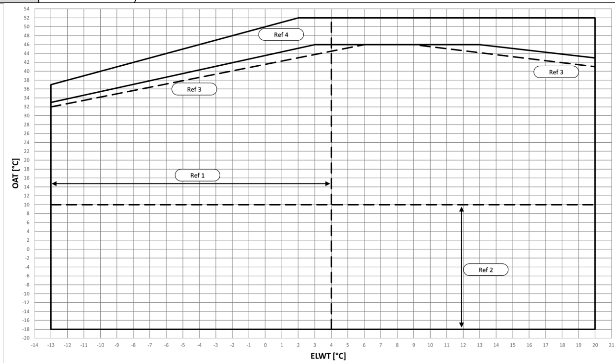
Fig. 3 – EWYTx0B-S Limitele Operationale ale Modulului de Racire
