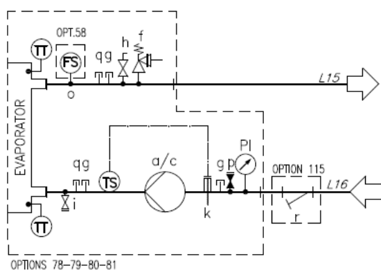
Рис. 18. Гидравлическая схема для одного насоса / двух насосов (компл. 78-79-80-81/134-135-136-137) (макс. рабочее давление 6 бар)
