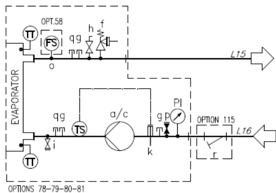
Obr. 18 – Hydraulická schéma samostatného čerpadla/dvojitého čerpadla (opt. 78-79-80-81/134-135-136-137) (max. prevádzkový tlak 6 barov)
