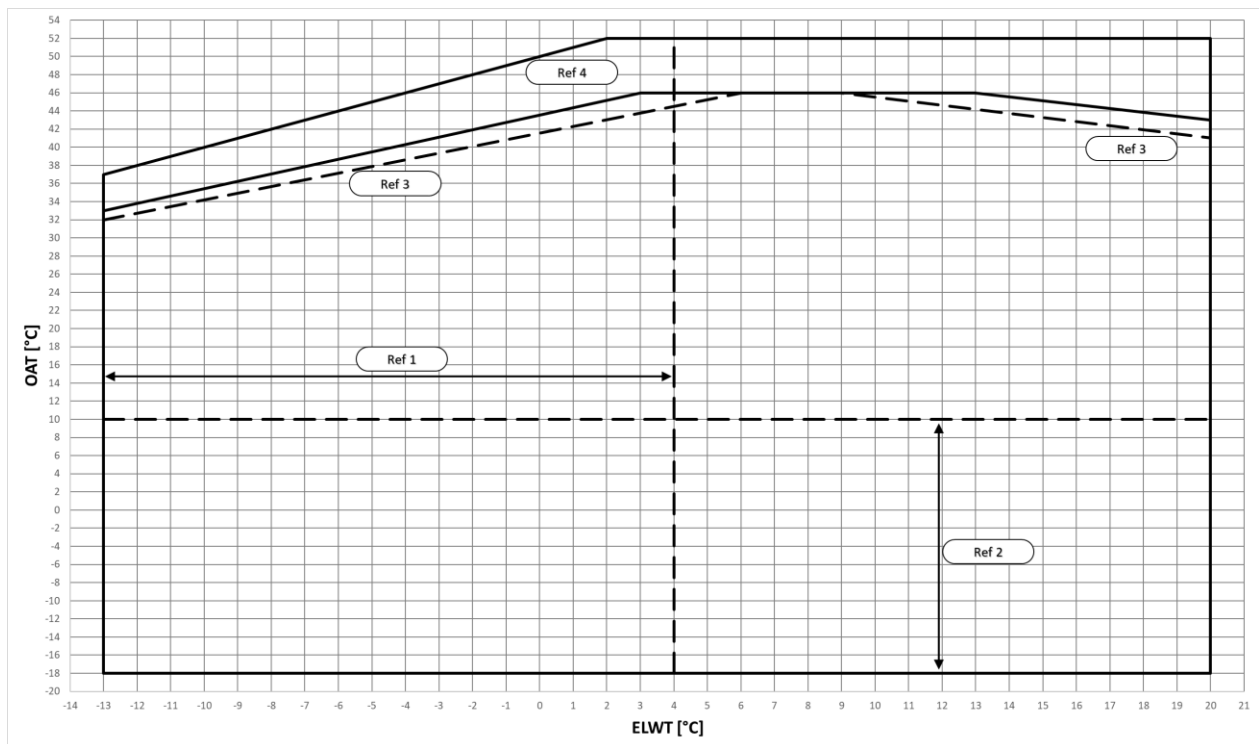
Obr. 3 – Prevádzkové limity režimu chladenia EWYTx0B-S
