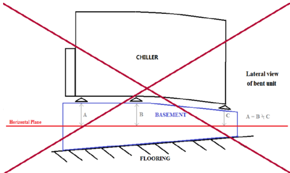
Obr. 10 – Vyrovnávanie jednotky
