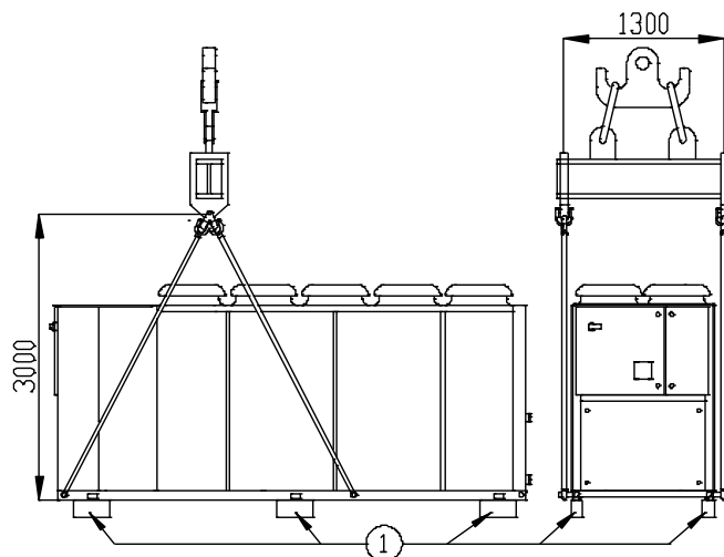
Enota s 4 dvignimi točkami
