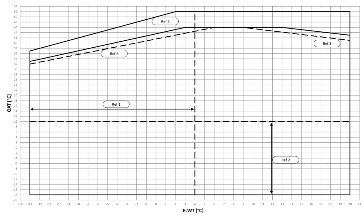
Fig. 3 – EWYTxx0B-S Operativa gränser för kylningsläge
