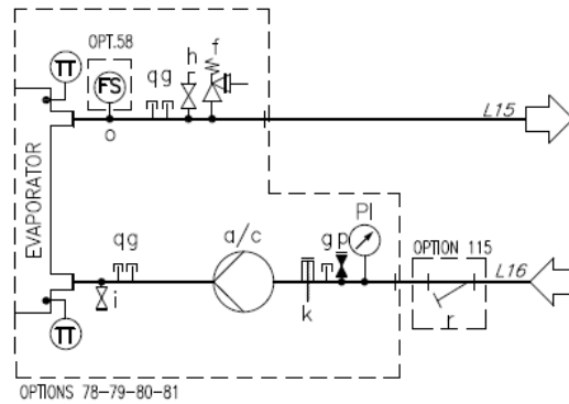
Fig. 15 – Hydrauliskt diagram för enkelpump / dubbelpump (EWYTxx5B) (alt. 78-79) (max arbetstryck 6 bar)
