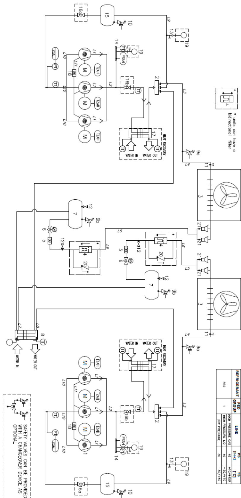
Fig. 21 – EWYTxx0B Kylkretsdiagram
