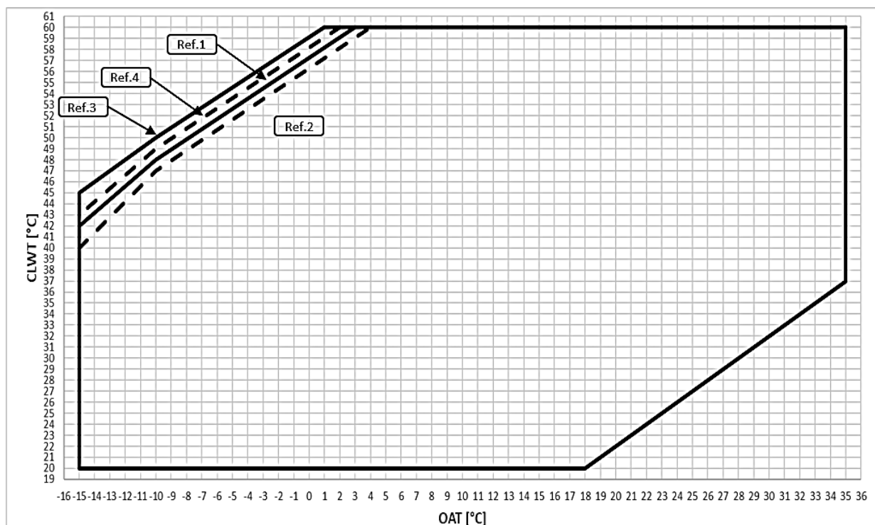
Фиг.° 8 - EWYT~B-X - OP.204 Работни граници в режим на отопление
