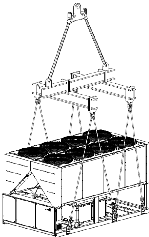
Агрегат с 6 точки за повдигане
