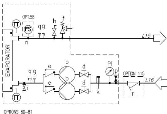
Фиг.° 17 - Хидравлична схема за двойна помпа (EWYTx5B) (опт. 80-81/136-137) (максимално работно налягане 6 bar)
