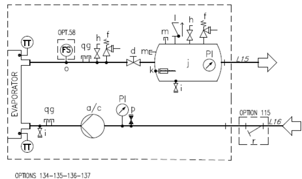
Фиг.° 16 - Хидравлична схема за единична помпа/двойна помпа с резервоар (EWYTx5B) (опт. 134-135) (максимално работно налягане 6 bar)
