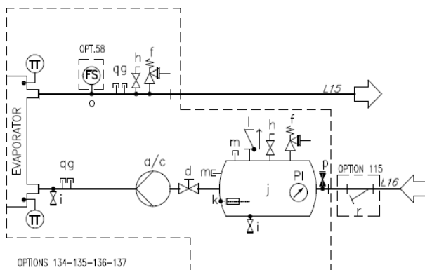
Фиг.° 16 - Хидравлична схема за единична помпа/двойна помпа с резервоар (EWYTx5B) (опт. 134-135) (максимално работно налягане 6 bar)
