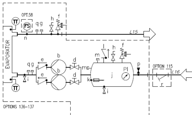
Фиг.° 17 - Хидравлична схема за двойна помпа (EWYTx5B) (опт. 80-81/136-137) (максимално работно налягане 6 bar)
