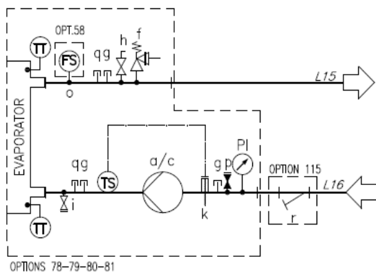
Фиг.° 18 - Хидравлична схема за единична помпа/двойна помпа (опт. 78-79-80-81/134-135-136-137) (максимално работно налягане 6 bar)
