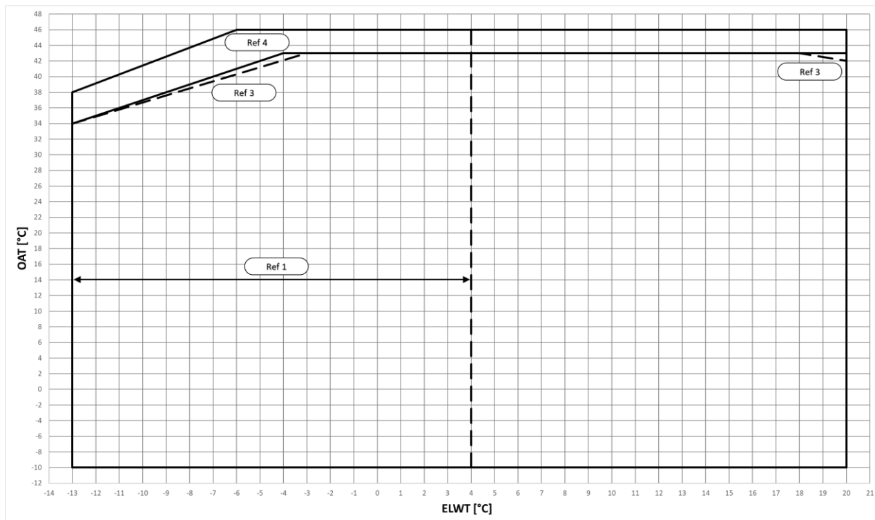
Фиг.°2 - Работни граници в режим на охлаждане на EWYTx5B-X
