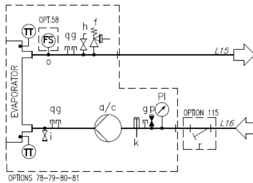
Фиг.° 15 - Хидравлична схема за единична помпа/двойна помпа (EWYTx5B) (опт. 78-79) (максимално работно налягане 6 bar)
