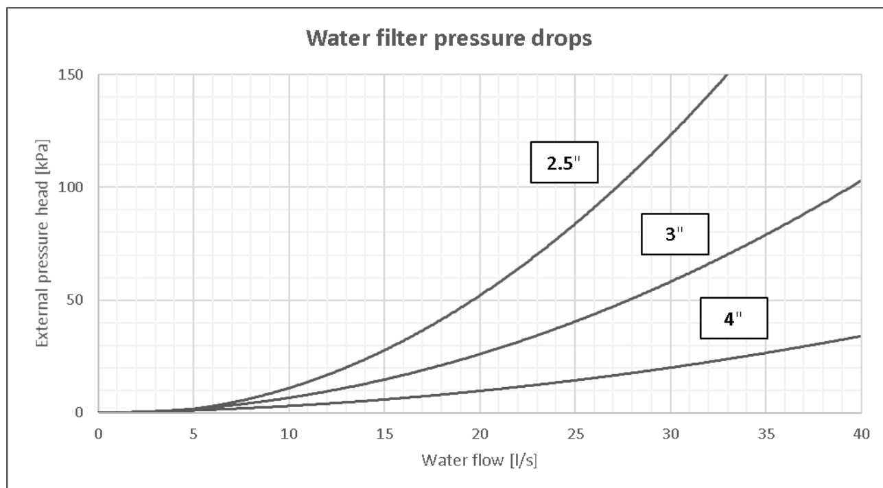
Фиг. ° 13 - Падане на налягането на водния филтър
