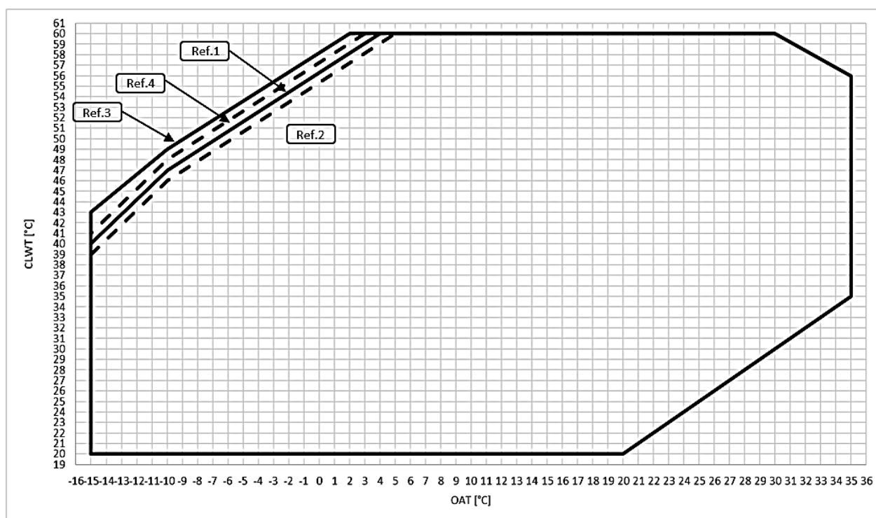
Фиг.° 7 - EWYT~B-S - OP.204 Работни граници в режим на отопление
