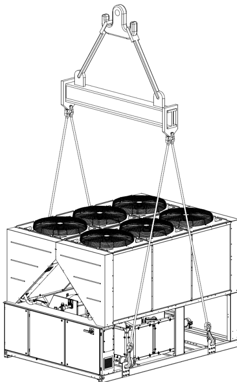
Агрегат с 4 точки за повдигане
