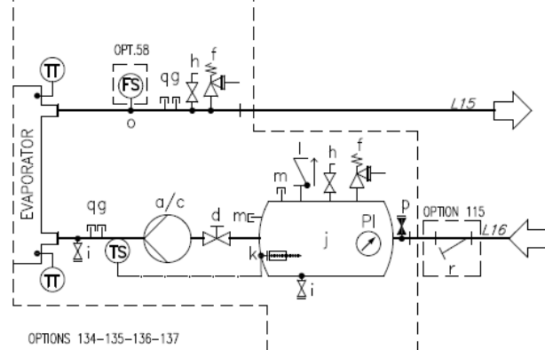
Фиг.° 18 - Хидравлична схема за единична помпа/двойна помпа (опт. 78-79-80-81/134-135-136-137) (максимално работно налягане 6 bar)
