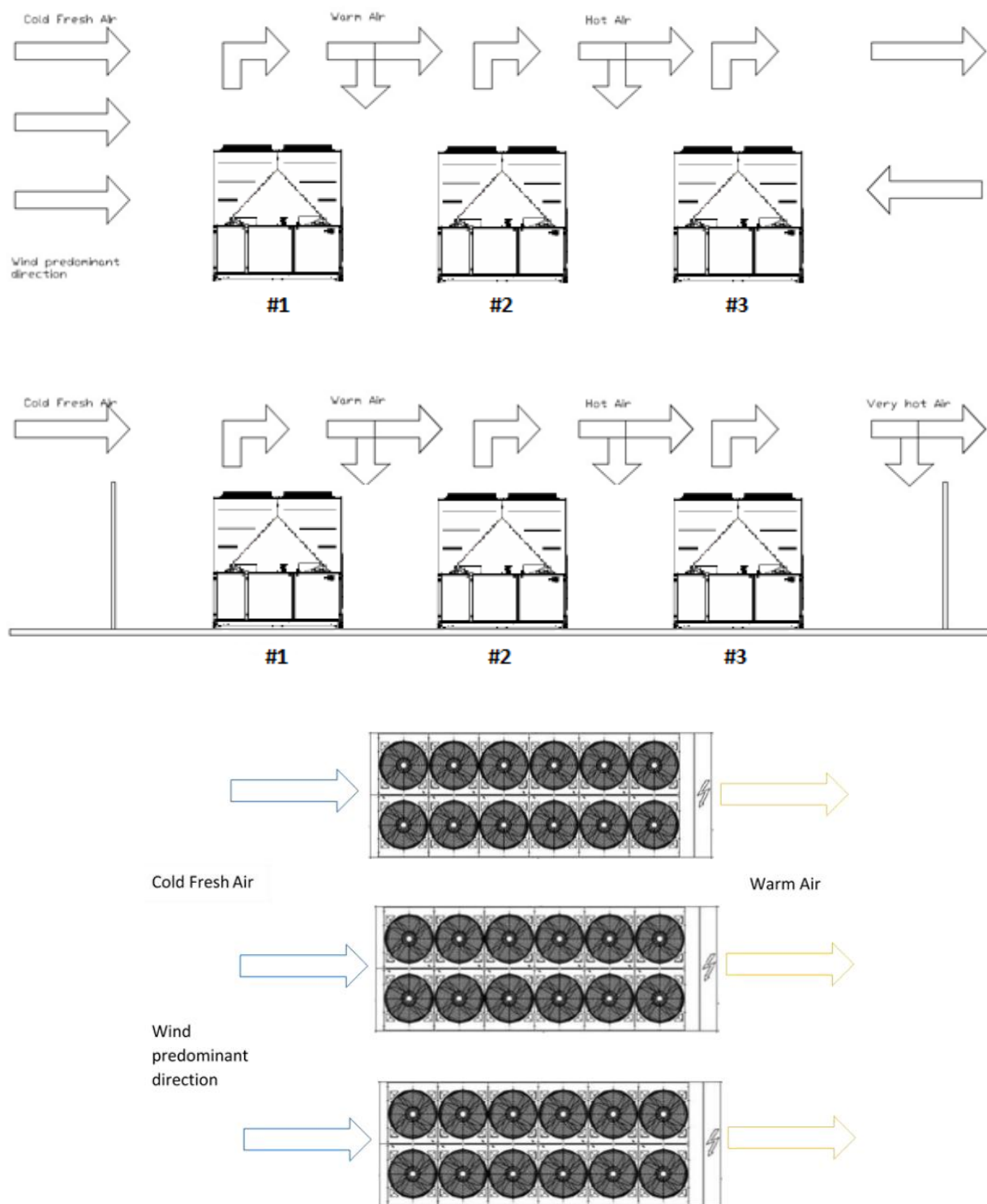
Фиг.° 12 - Монтаж на няколко агрегата (режим на охлаждане)
