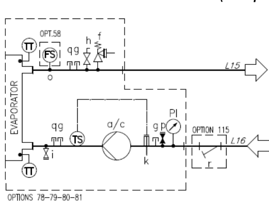
Obr. 17 – Hydraulické schéma pro dvojité čerpadlo (EWYTx5B) (vol. 80-81/136-137) (max. provozní tlak 6 bar)
