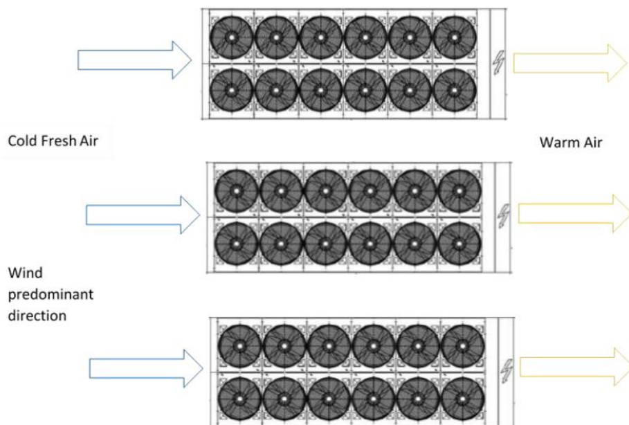
Abb. 12 – Installation mehrerer Geräte (Kühlbetrieb)
