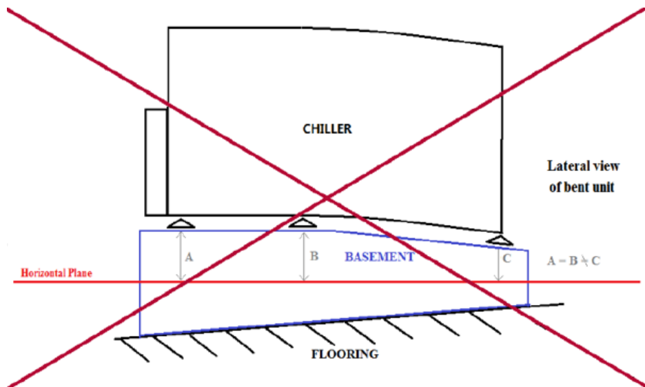
Abb. 10 – Ausrichtung des Geräts
