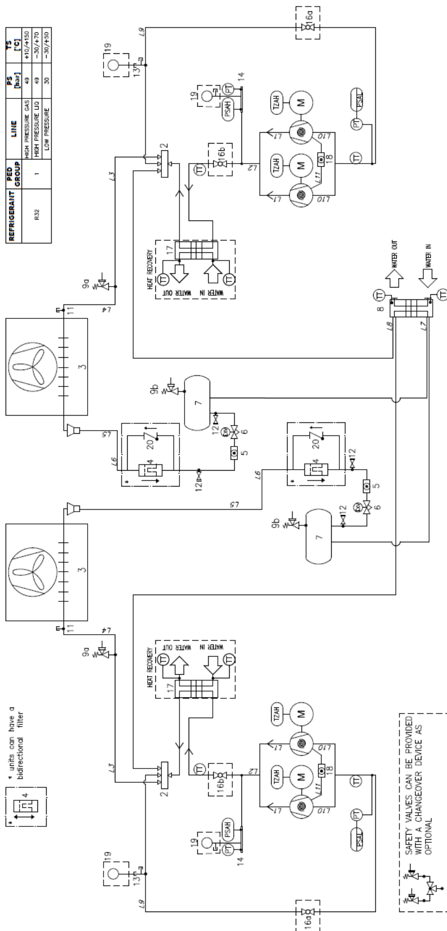
Fig. 20 – Unidad de circuito doble EWYTxx5B Diagrama de tubería de refrigerante (P&ID)
