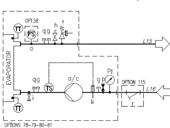
17. ábra – Dupla szivattyú hidraulikus diagramja (EWYTx5B) (opt. 80-81/136-137) (max. üzemi nyomás 6 bar)
