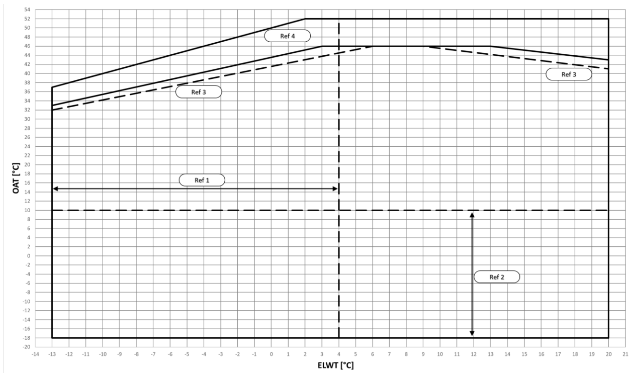
Fig. 3 – EWTxx0B-S Limitele Operationale ale Modulului de Racire
