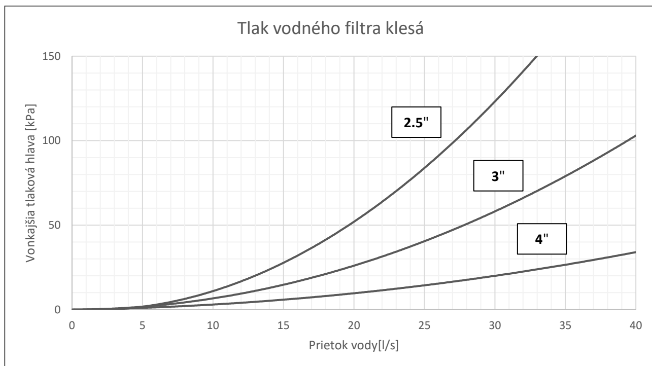
Obr. 13 – Pokles tlaku vodného filtra
