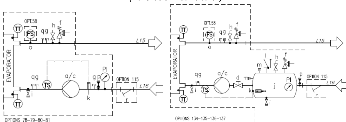
Slika 17 – Hidravlična shema za dvojno črpalko (EWYTx5B) (opc. 80-81/136-137) (maks. delovni tlak 6 barov)
