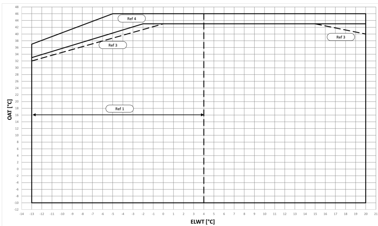
Slika 1 – EWYTx5B-S Delovne omejitve hladilnega načina
