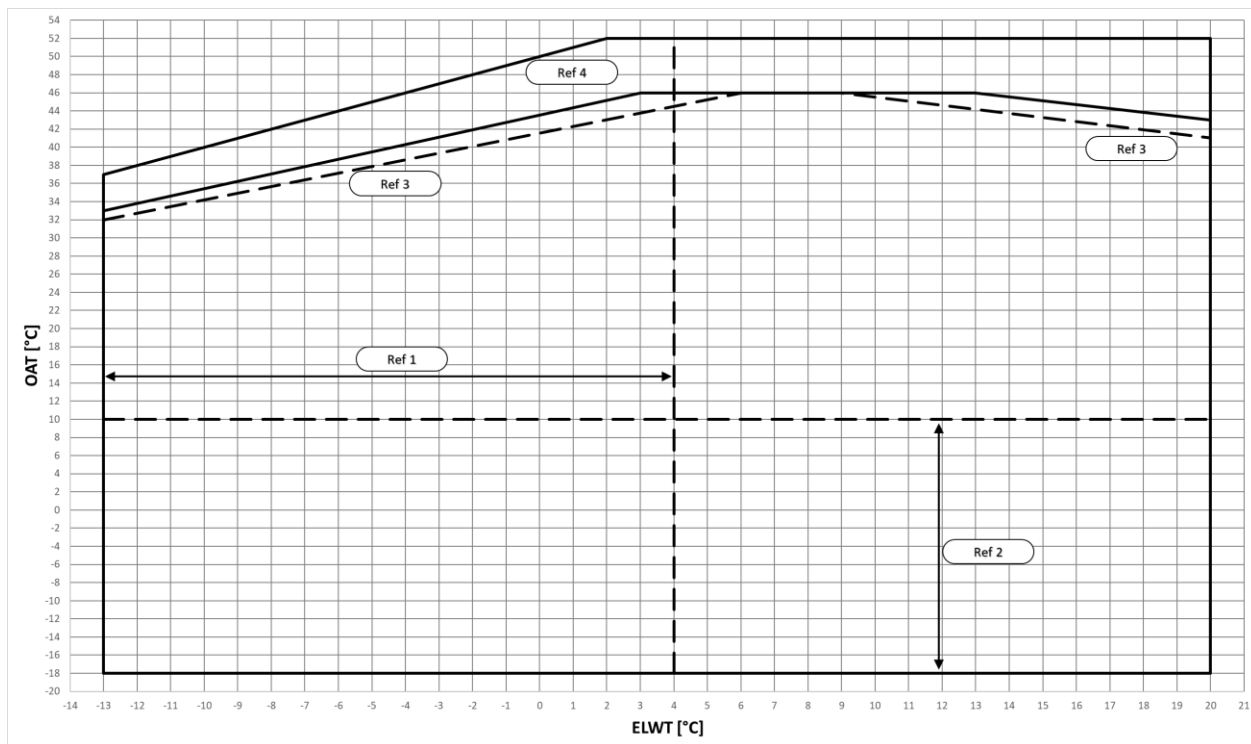
Slika 3 – EWYTxx0B-S Delovne omejitve načina hlajenja
