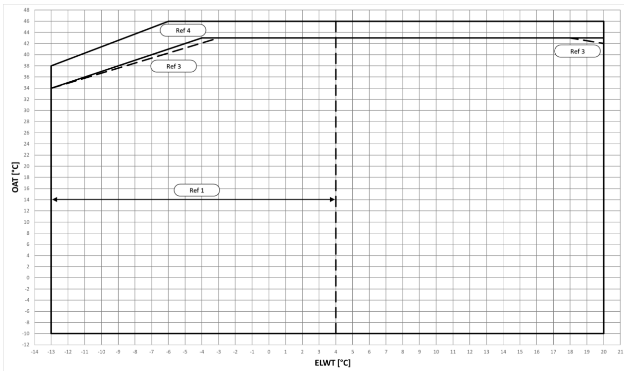
Slika 2 – EWYTxx5B-X Delovne omejitve načina hlajenja
