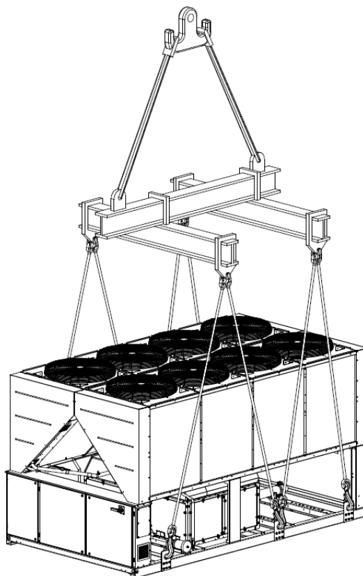
Enota s 6 dviznimi točkami
