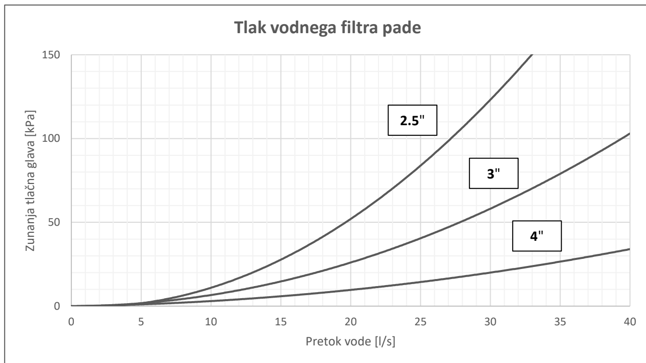
Slika 13 – Padec tlaka vodnega filtra
