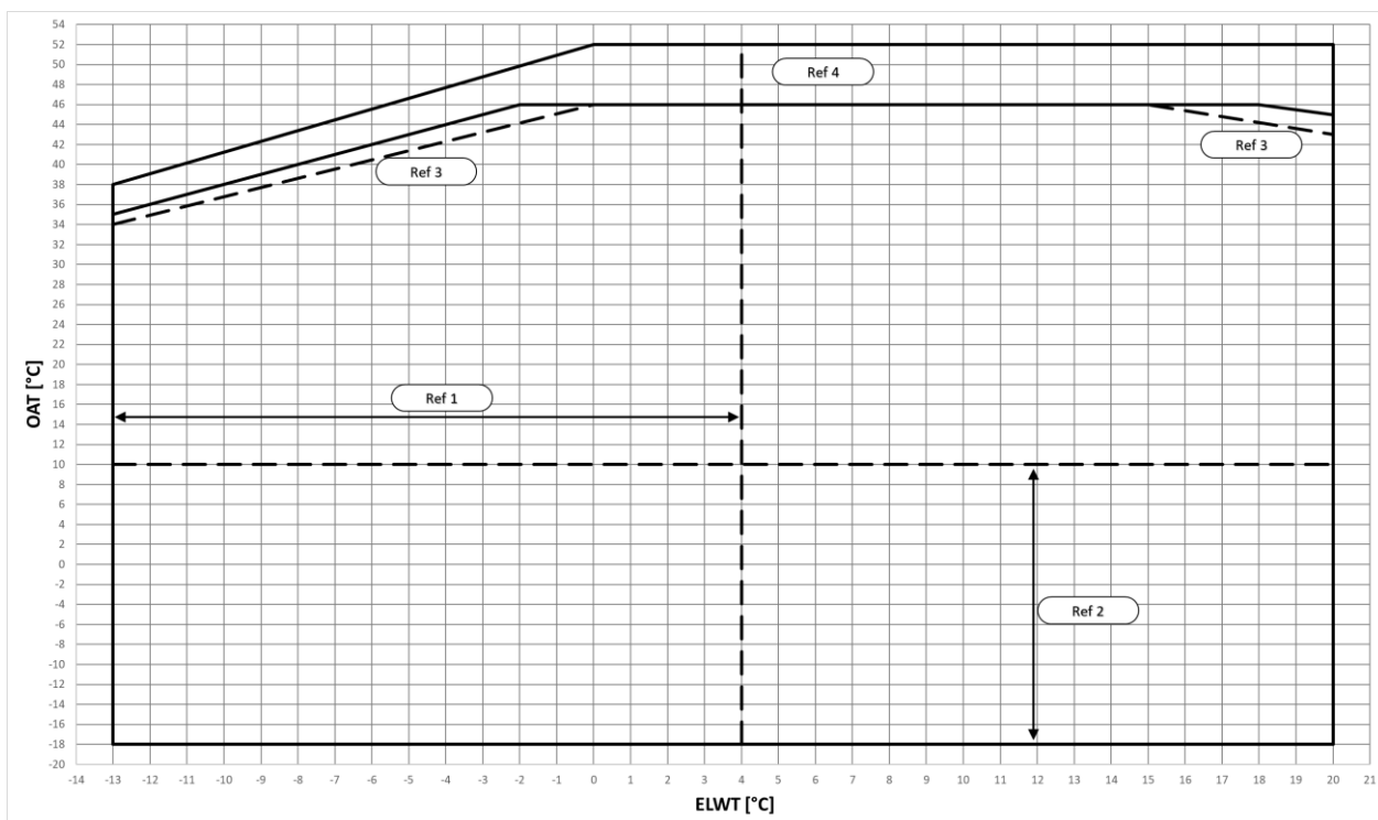
Slika 4 – EWYTx0B-X Delovne omejitve načina hlajenja
