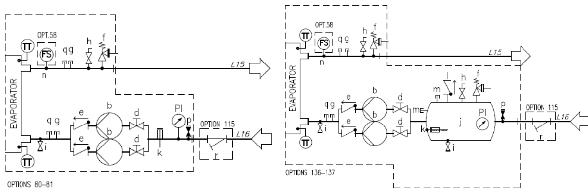
Fig. 17 – Hydrauliskt diagram för dubbelpump (EWYTx5B) (alt. 80-81/136-137) (max arbetsstryck 6 bar)
