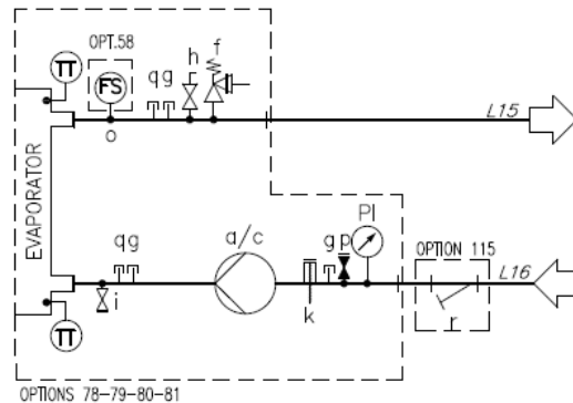
Fig. 15 – Hydrauliskt diagram för enkelpump / dubbelpump (EWYTx5B) (alt. 78-79) (max arbetsstryck 6 bar)
