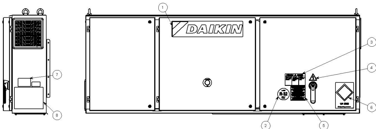
Fig. 23 – Beskrivning av märkningarna applicerade på elpanelen EWYTxx0B
