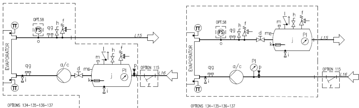
Fig. 16 – Hydrauliska schema för enkelpump / dubbelpump med tank (EWYTx5B) (alt. 134-135) (max arbetsstryck 6 bar)
