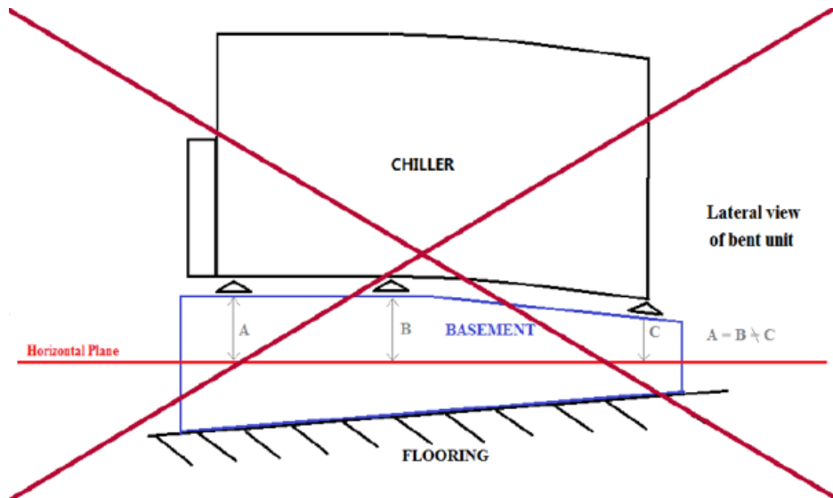
Fig. 10 – Utplaning av enhet
