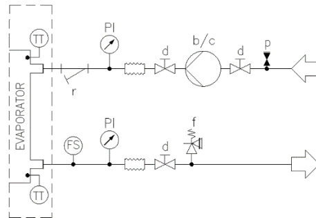
Fig. 14 – Hydrauliskt diagram utan pump(ar) ombord (max. arbetsstryck 20 bar)
