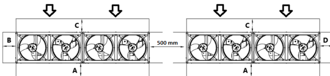
Figura 7 –Unidades instaladas lado-a-lado ao longo dos lados mais curtos, B ou D
