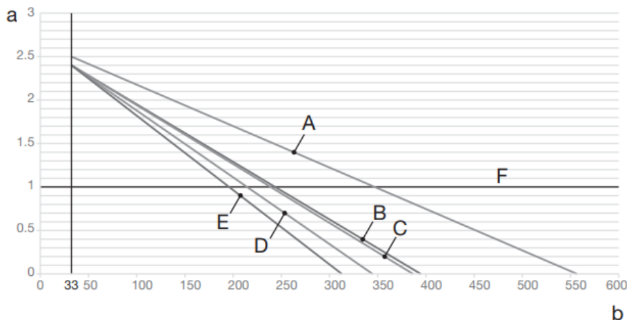
Figura 17 - Pressão inicial do vaso de expansão com base no volume máximo de água
