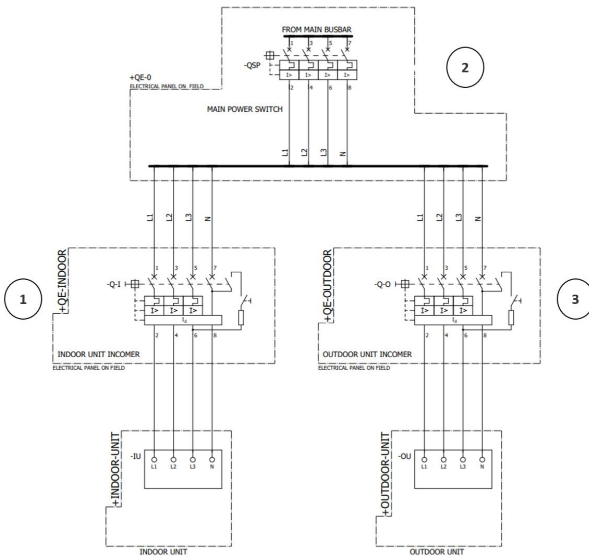
20. ábra – Fő huzalozási rajz
