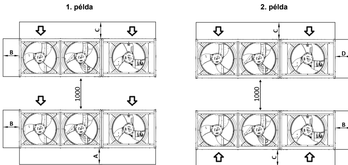
11. ábra – Hosszú oldaluk (1. vagy 2. példa) mentén egymás mellé telepített egységek
