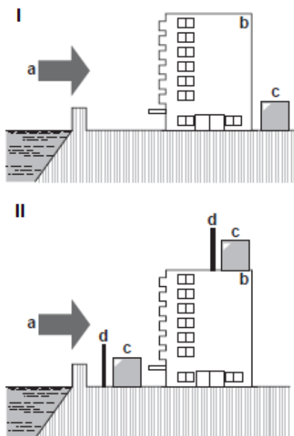
Abbeeldingen 11 – Installatie van de buitenunit aan zee
