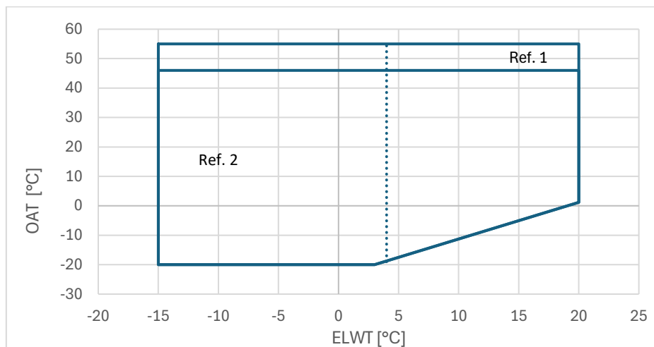
Afbeeldingen 1 - werkingssbereik koeling EWYE-CZ
