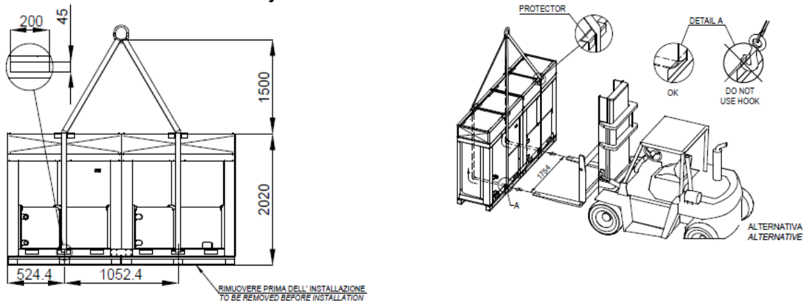
Afbeeldingen 4 – Het heffen van het DUAL-systeem
